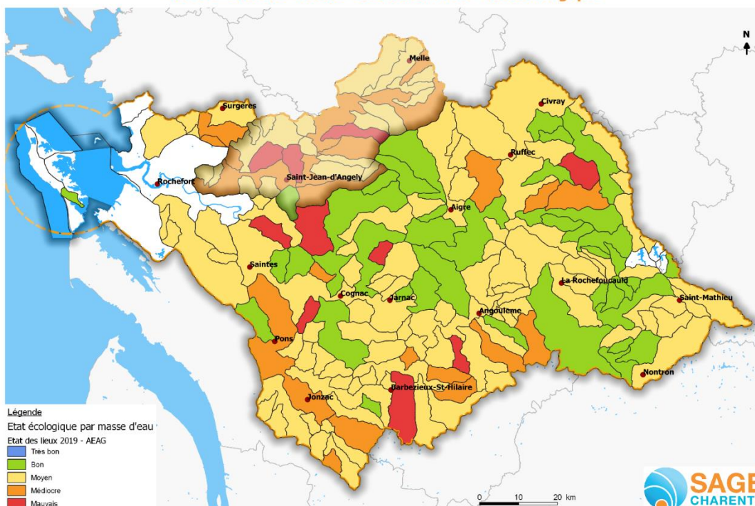
IG.5.1 - Etat des masses d'eau de surface - Etat écologique
