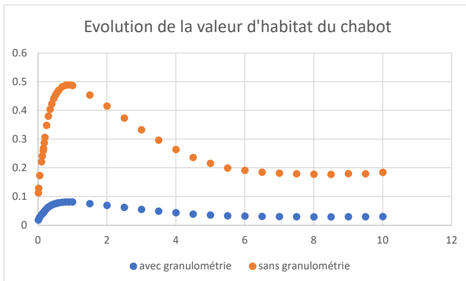
Figure 55 : Evolution sans granulométrie (en orange) et avec granulométrie (en bleu) de la valeur d'habitat pour le chabot sur toute la gamme de débit
