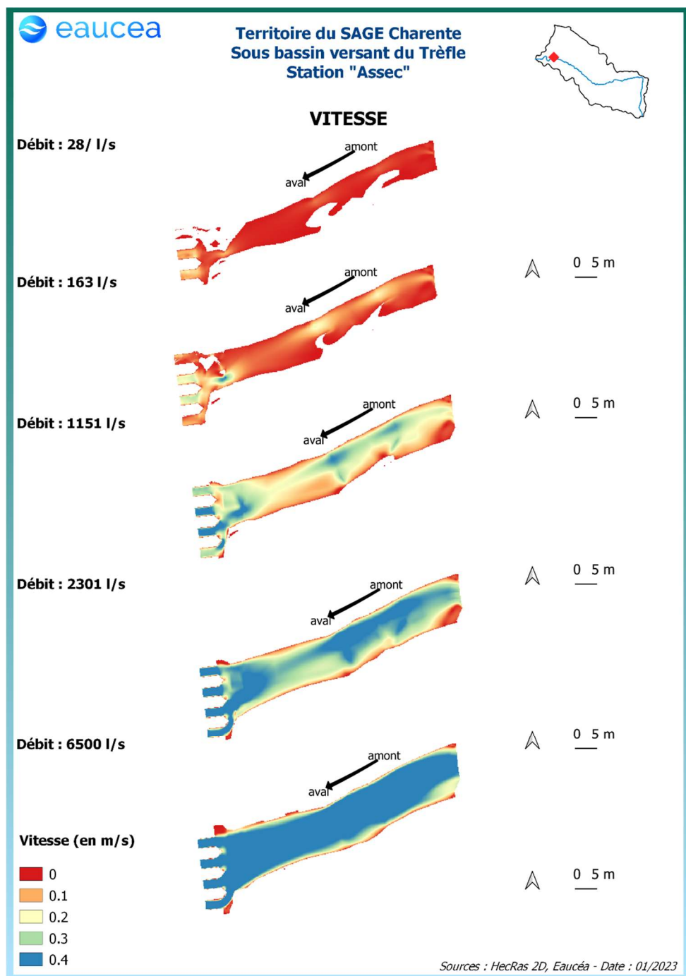
Figure 47: Evolution des vitesses d'écoulement sur la station du Pont d'Usseau à différents débits
