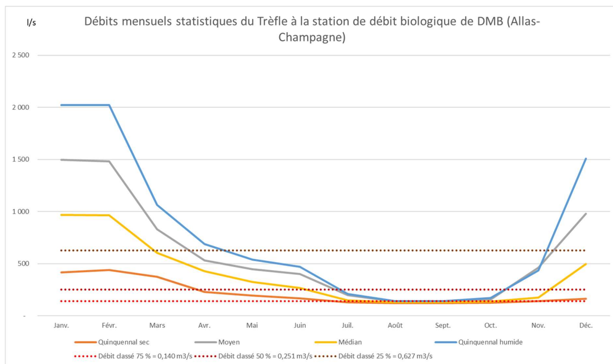
Figure 9 : Débits mensuels statistiques et débits classés du Trèfle au Pont d'Usseau (station « Assec »)
