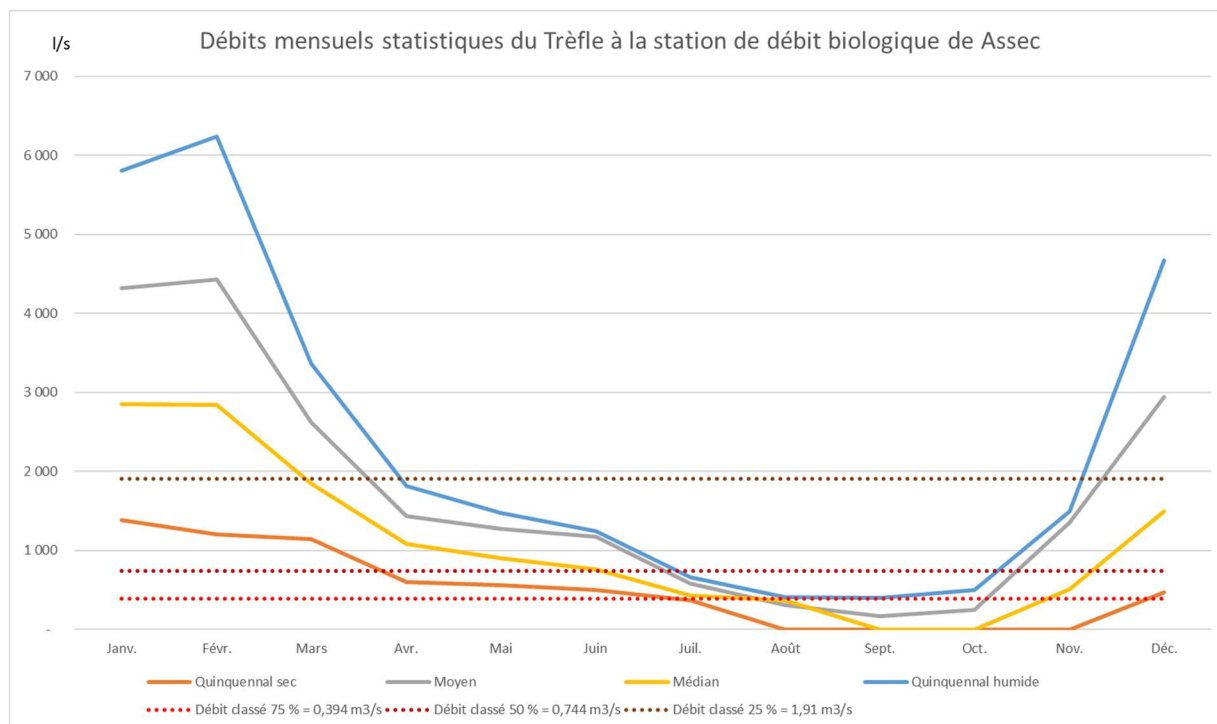
Figure 11 : Débits mensuels statistiques et débits classés du Trèfle au Pont d'Usseau (station « Assec »)
