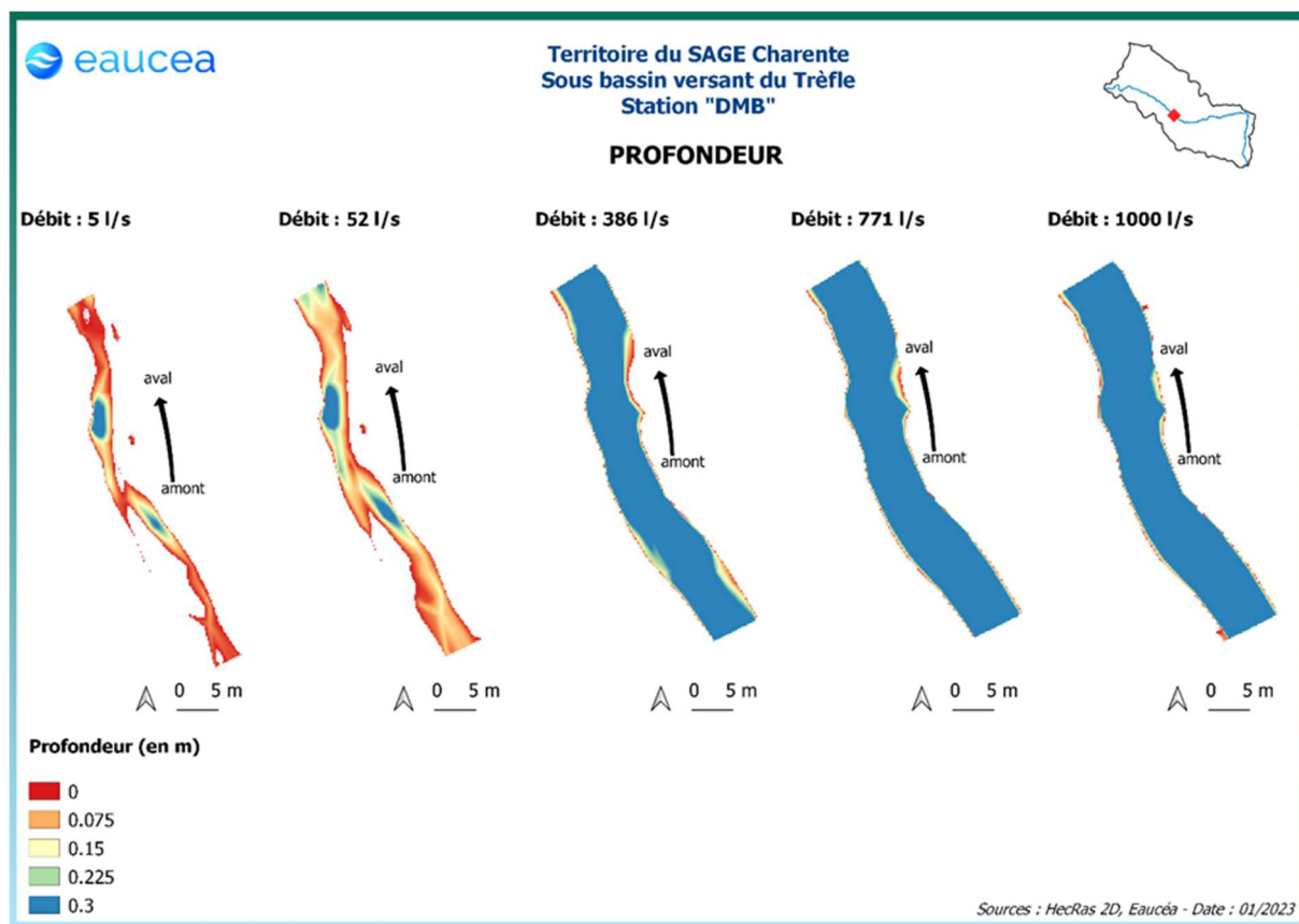
Figure 23: Evolution des profondeurs sur la station DMB à différents débits
