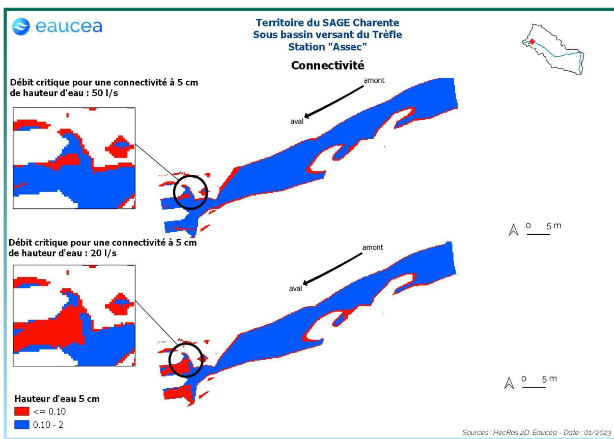
Figure 52: Connectivité de la station du Pont d'Usseau pour un seuil de 5 cm de hauteur d'eau
