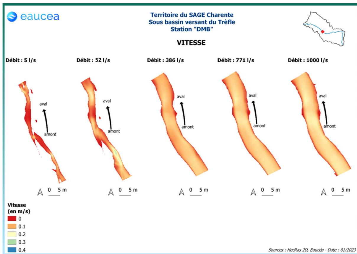
Figure 24: Evolution des vitesses d'écoulement sur la station DMB à différents débits
