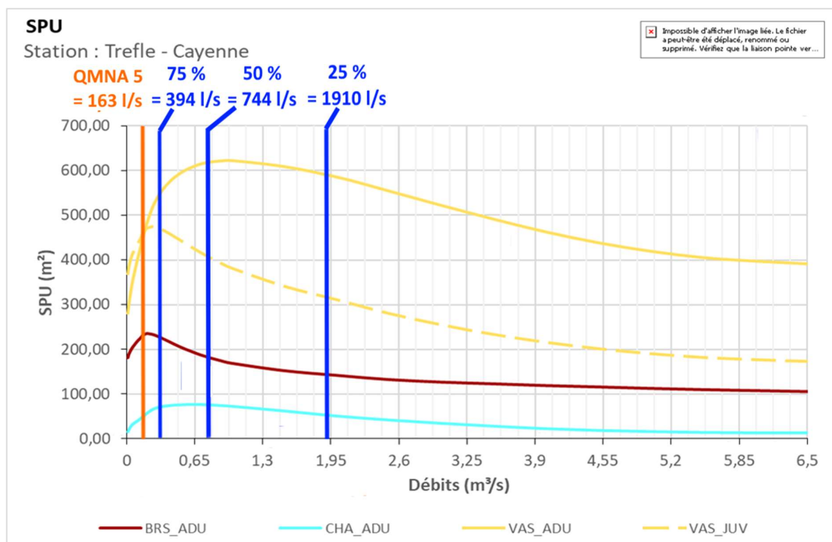
Figure 57: Surfaces pondérées utiles des différents stades du brochet, du vairon et du chabot de la station du Pont d'Usseau
