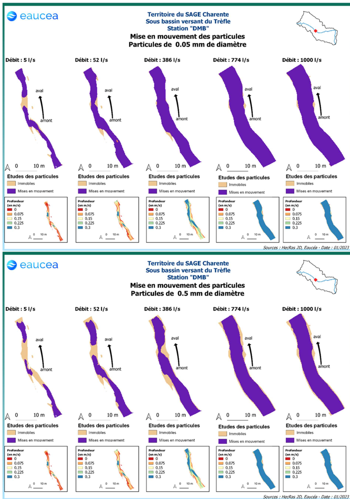
Figure 27 : Mise en mouvement des particules fines sur la station d'Allas-Champagne
