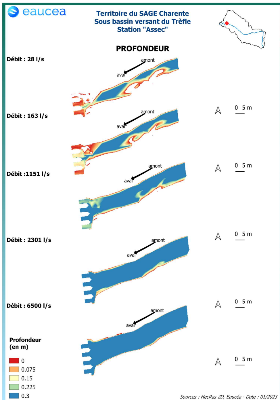
Figure 46: Evolution des profondeurs sur la station du Pont d'Usseau à différents débits
