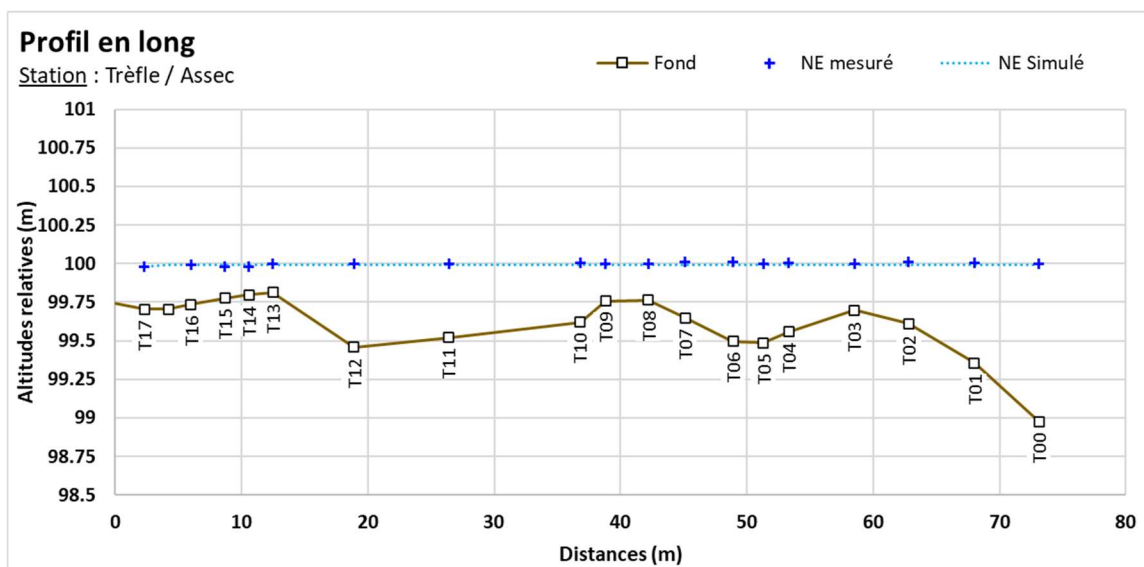
Figure 41 : Profil en long de la station et comparaison des niveaux d'eaux simulé et mesuré
