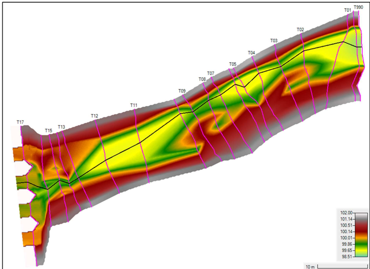
Figure 39 : Maillage de calcul et topographie de la station Assec - Trèfle
