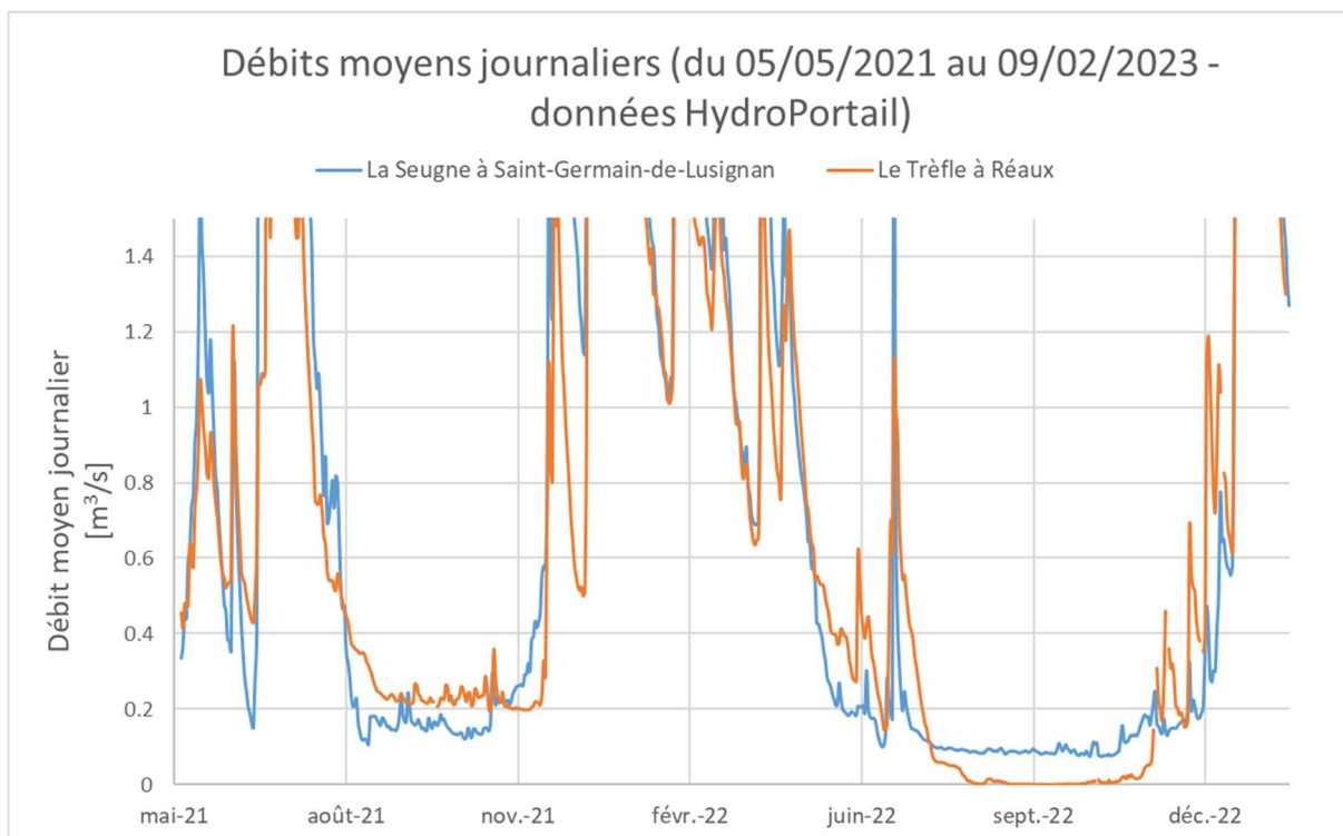
Figure 3: Hydrogrammes observés aux stations du Trèfle à Réaux et de la Seugne à Saint-Germain-de-Lusignan – zoom basses eaux
