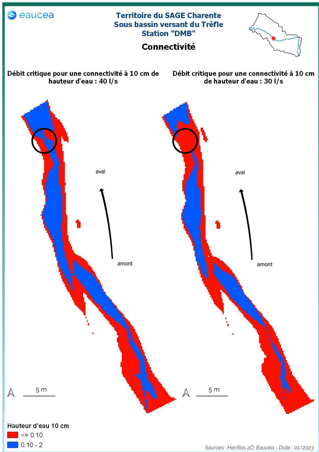
Figure 30: Connectivité de la station sur le Trèfle pour un seuil de 10 cm de hauteur d'eau
