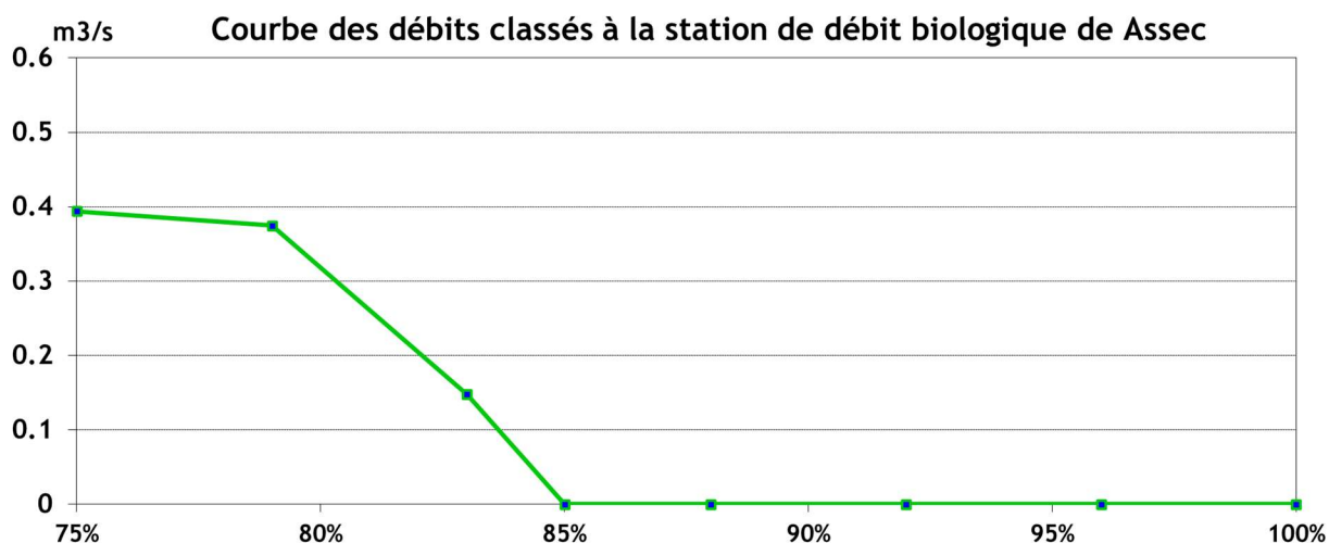
Figure 8: Domaine des étiages : Courbe des débits journaliers classés en période de basses-eaux du Trèfle à la Cayenne (Pont d'Usseau)
