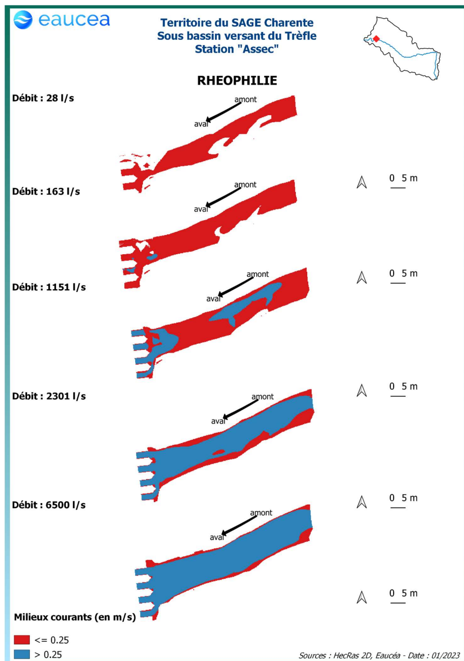
Figure 48: Evolution des milieux courants sur la station du pont d'Usseau
