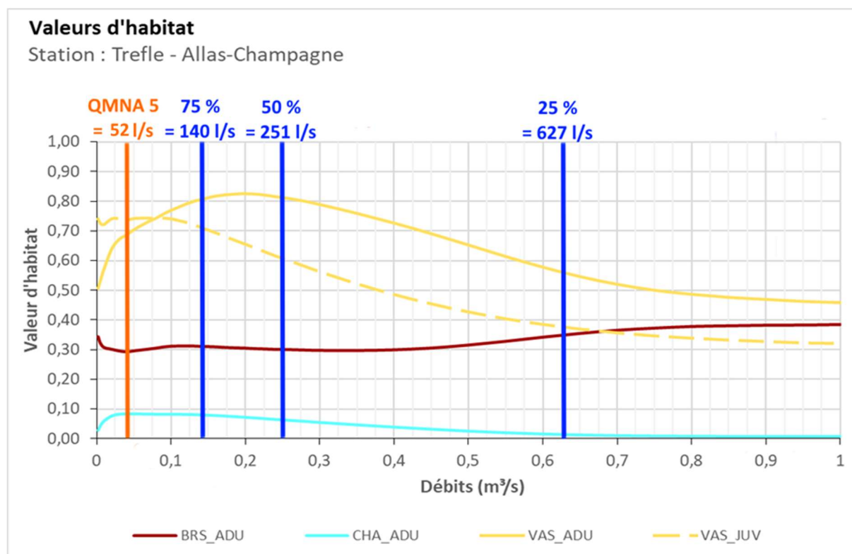
Figure 31: Valeurs d'habitat des différents stades du brochet, du vairon et du chabot de la station DMB
