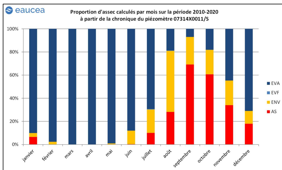
Figure 43 : Répartition mensuelle des intensités d'assec calculées à partir de la chronique piézométrique mesurée au piézomètre 07314X0011/S
