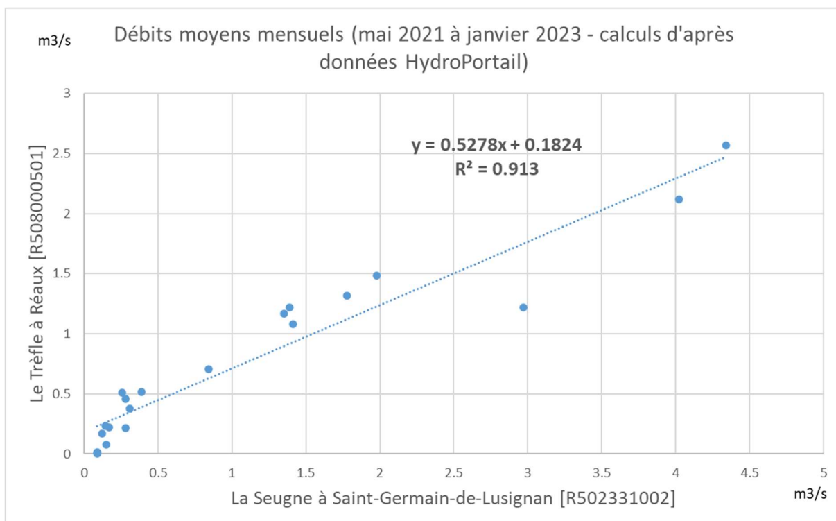
Figure 4: Relation entre les débits moyens mensuels des stations du Trèfle à Réaux et de la Seugne à Saint-Germain-de-Lusignan
