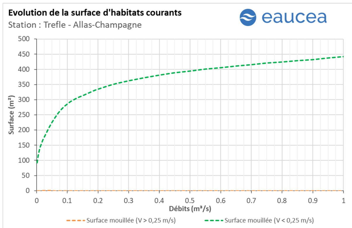
Figure 26 : Evolution de surface lotique (orange) et lentique (vert)
