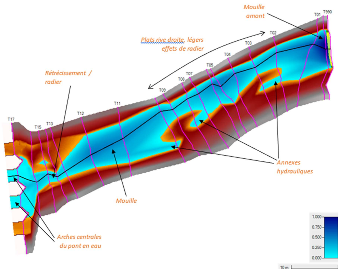
Figure 40 : Faciès d'écoulements du modèle (fidèles aux observations de terrain) et profondeur (en mètre)
