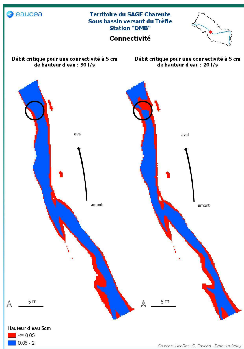
Figure 29: Connectivité de la station DMB pour un seuil de 5 cm de hauteur d'eau
