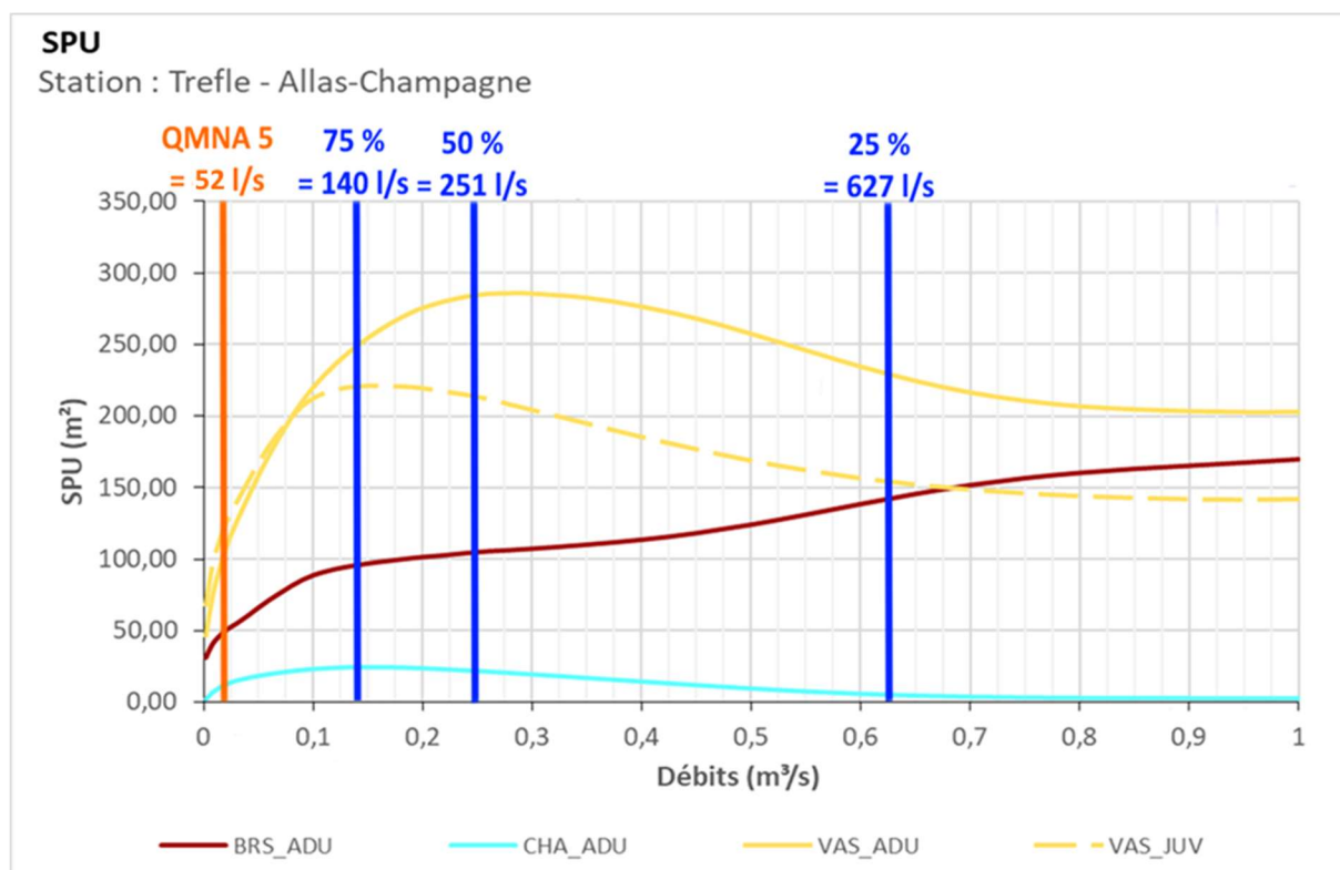
Figure 33: Surfaces pondérées utiles des différents stades du brochet, du vairon et du chabot de la station DMB
