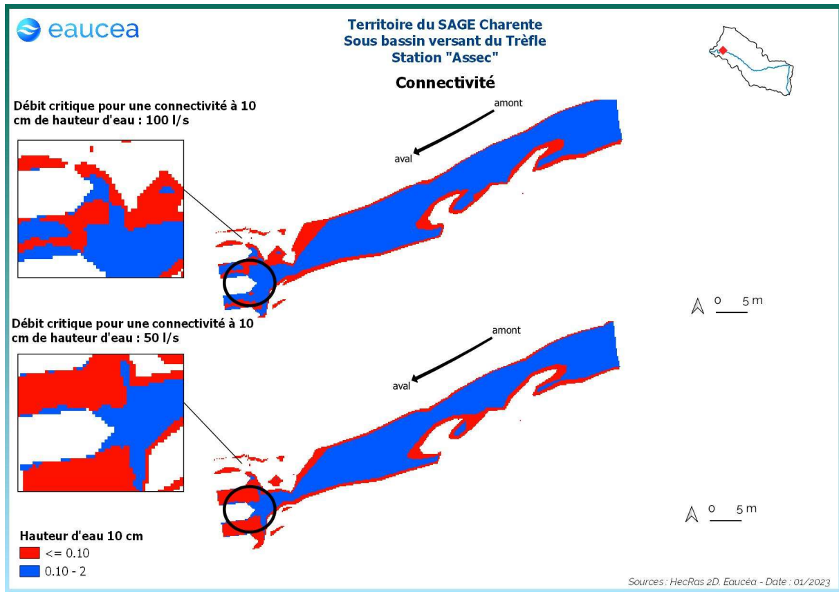
Figure 53: Connectivité de la station sur le Trèfle pour un seuil de 10 cm de hauteur d'eau
