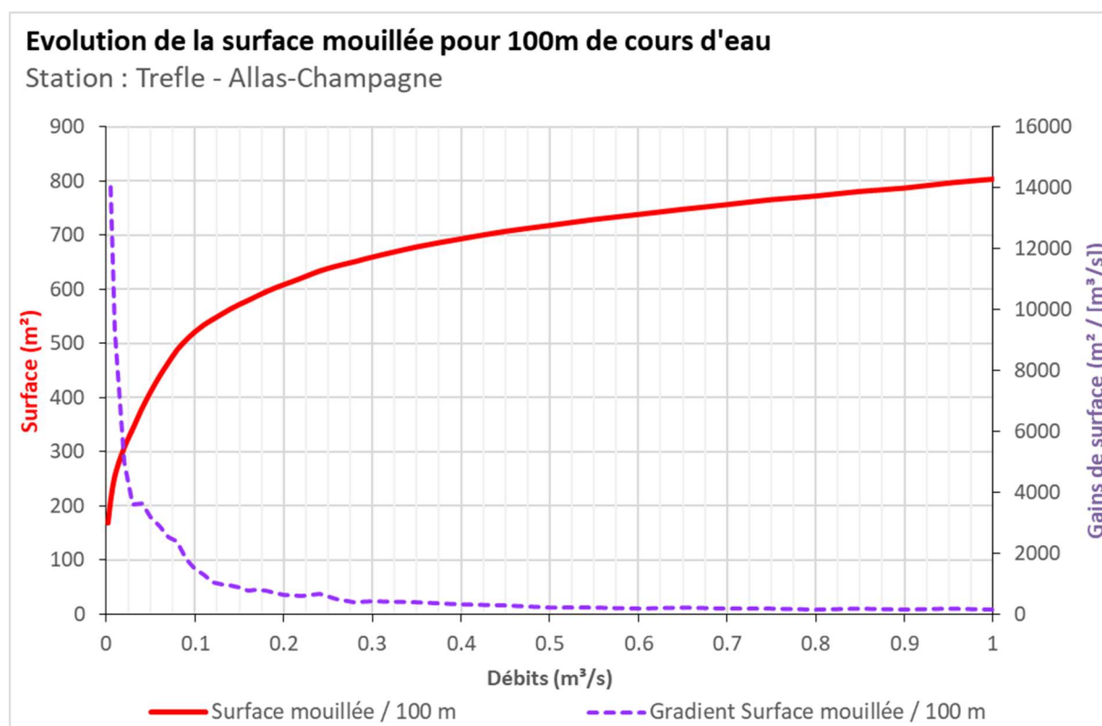
Figure 21 : Evolution de la surface mouillée à Allas-Champagne
