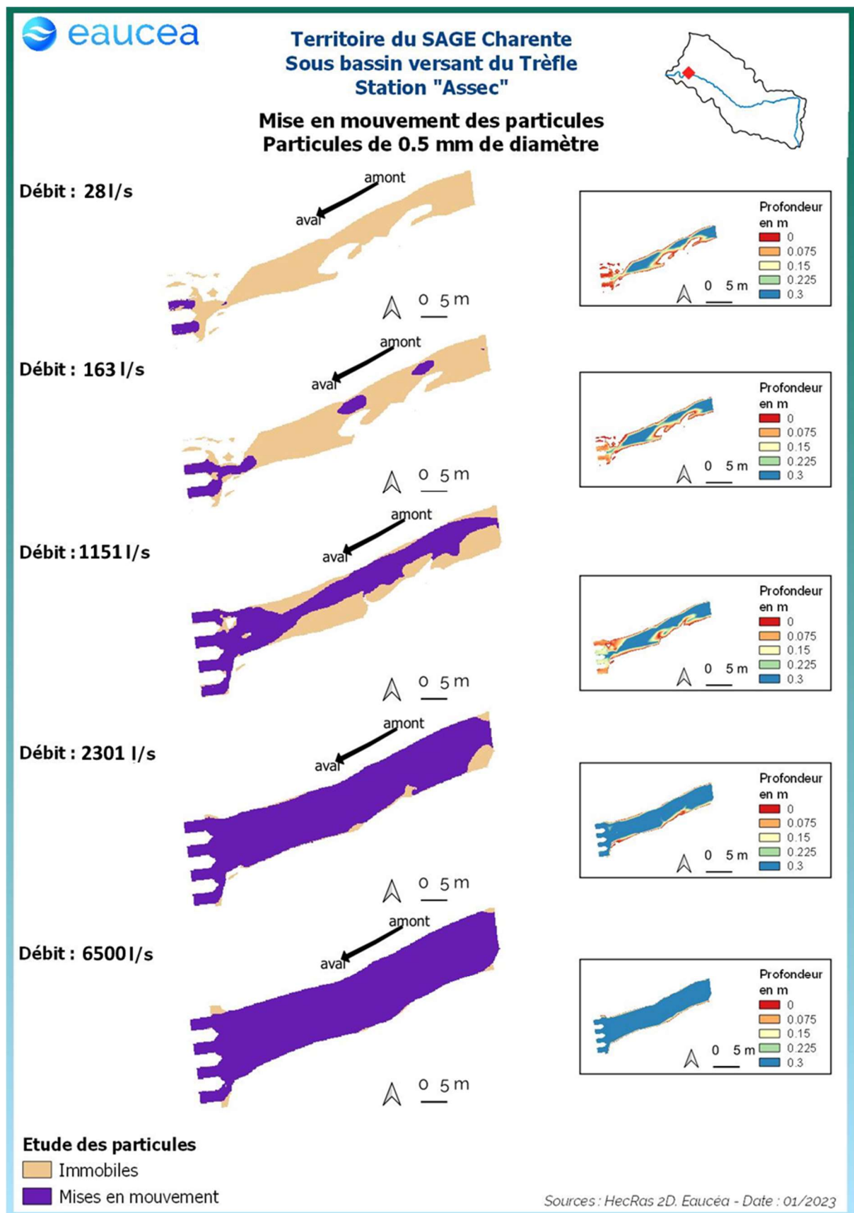
Figure 50 : Mise en mouvement des particules fines sur la station du Pont d'Usseau
