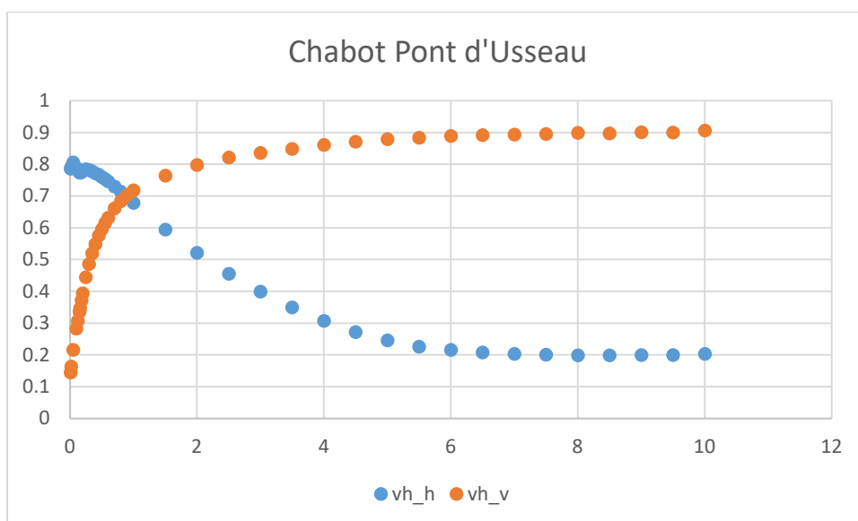
Figure 56 : Evolution des composantes "vitesse" (en orange) et "hauteur d'eau" (en bleu) de la valeur d'habitat pour le chabot sur toute la gamme de débit
