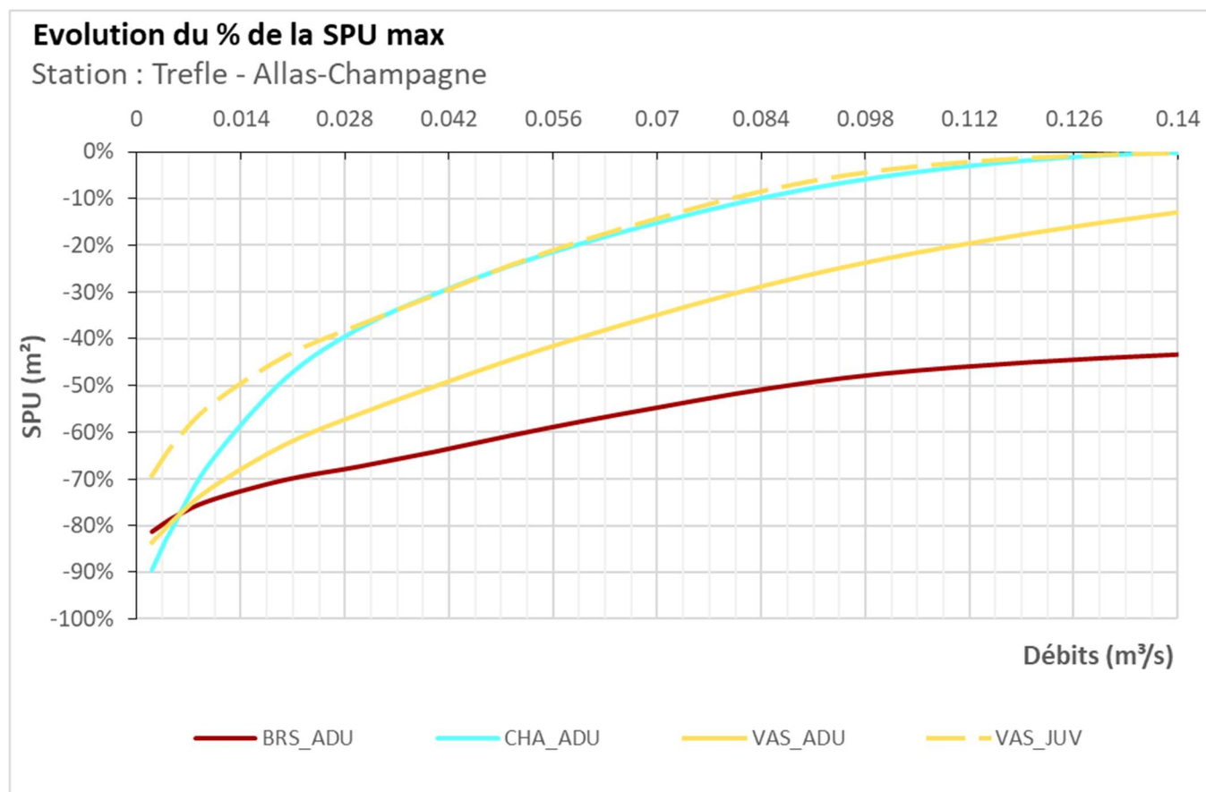
Figure 35 Zoom sur l'étiage du % des surfaces pondérées utiles maximales des différents stades du brochet, du vairon et du chabot de la station DMB
