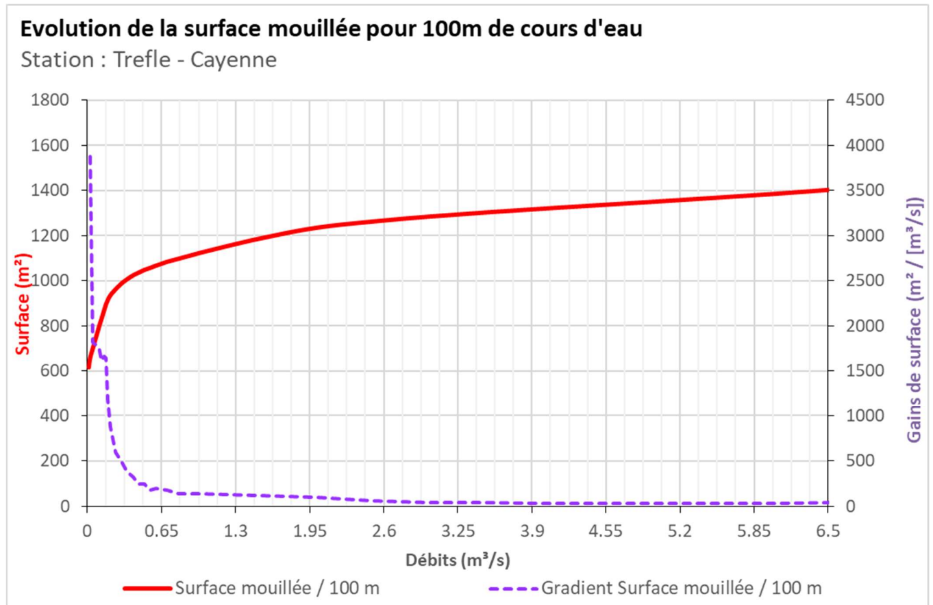
Figure 44 : Evolution de la surface mouillée au Pont d'Usseau
