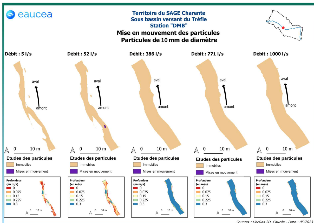
Figure 28 Mise en mouvement des particules grossières sur la station d'Allas-Champagne
