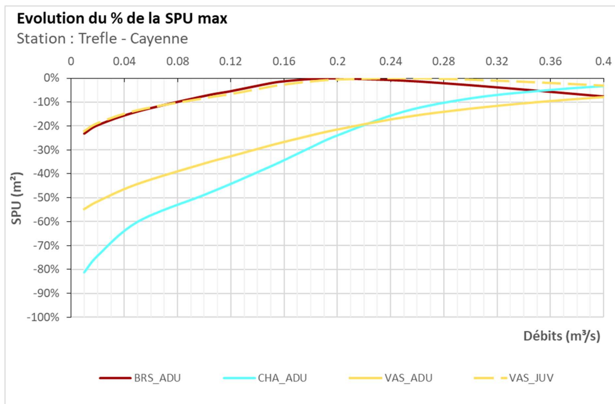
Figure 59 zoom sur l'étiage du % des surfaces pondérées utiles maximales des différents stades du brochet, du vairon et du chabot de la station du Pont d'Usseau
