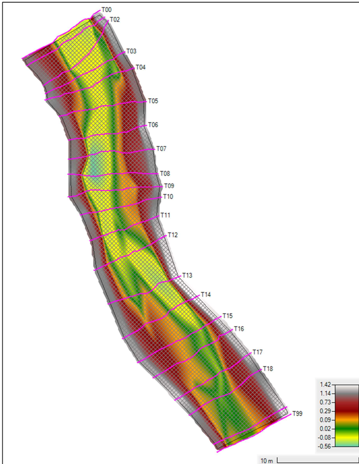
Figure 18 : Maillage de calcul et topographie de la station modélisée
