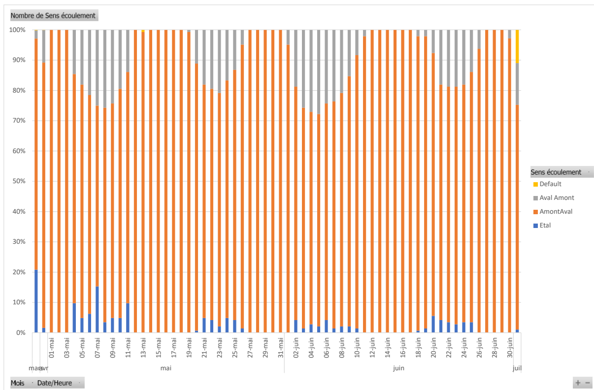
Figure 30: Sens d'écoulement au barrage en fonction des hauteurs d'eau amont et aval sur mai et juin
