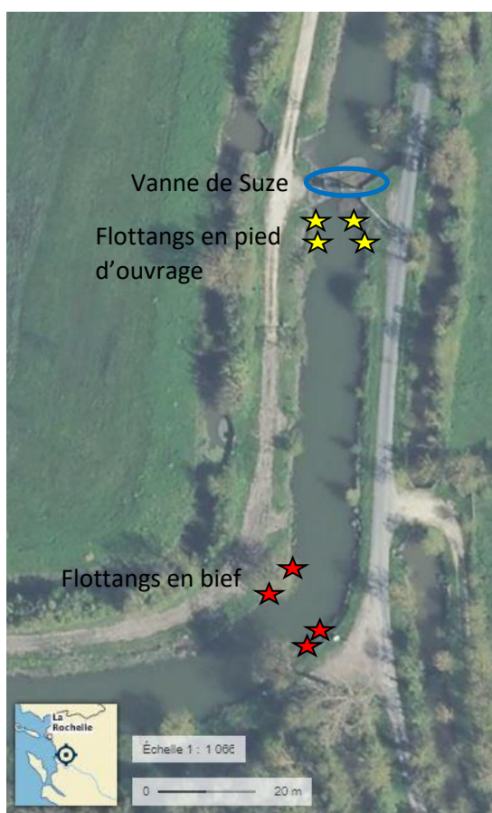
Figure 38 : Site de Suze et disposition des flottangs
