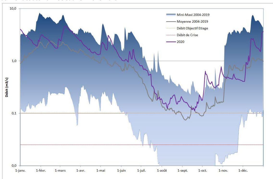
Figure 11 : Les débits à St André de Lidon sur la Seudre en 2020
