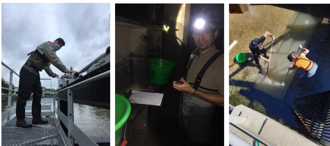
Figure 26 : Photos des sessions de piégeage : fermeture vanne, mesure de nuit, récupération des poissons de jour
