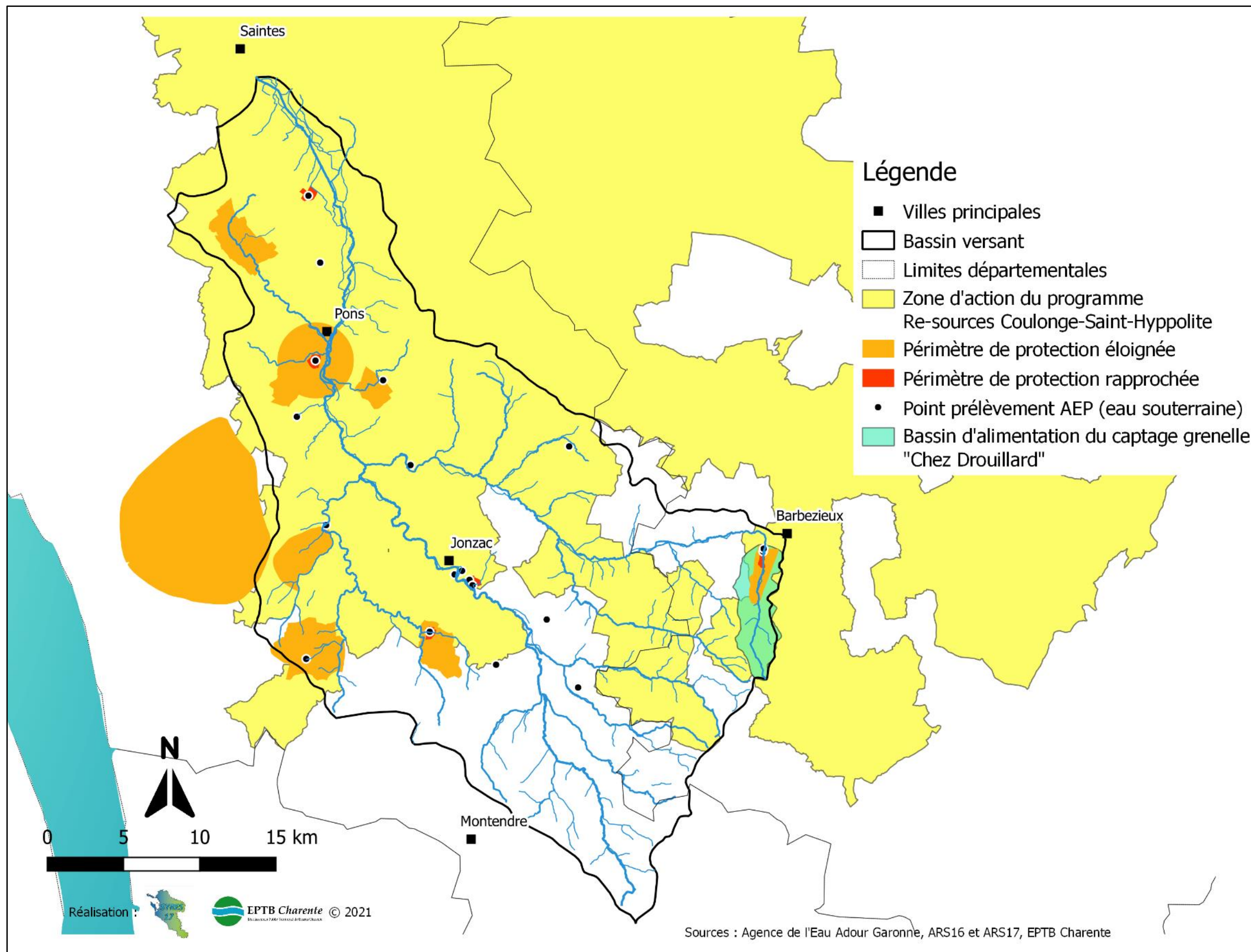
Carte 15 : Zones bénéficiant d'un statut de protection lié à la reconquête de la qualité de l'eau
