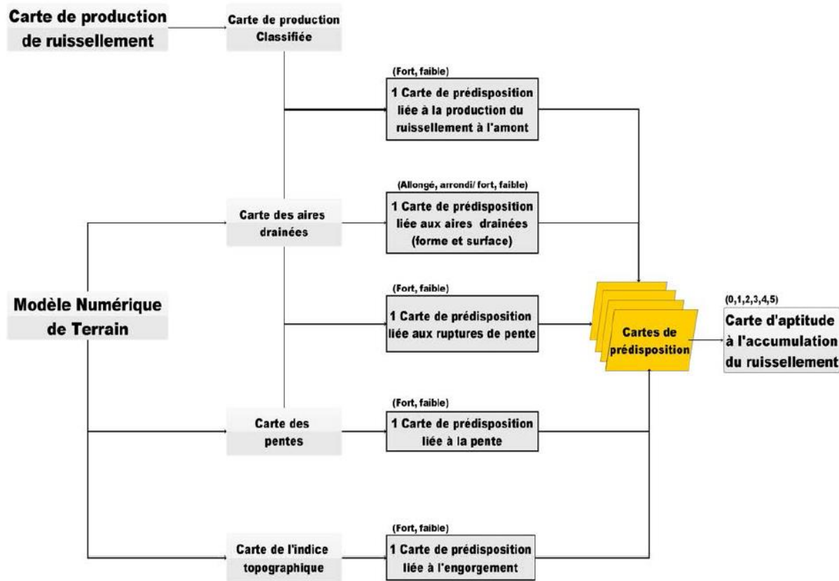
Figure 19 : Etablissement de la CAC (source : DEHOTIN J., BREIL P. Projet IRIP : Rapport technique Cartographie de l'aléa ruissellement. Note Méthodologique. Juillet 2011 ; p23)
