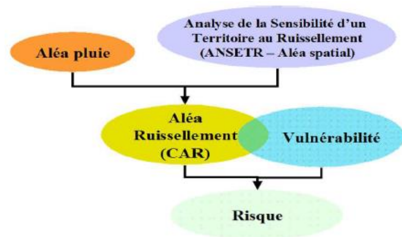
Figure 3 : Principe de la méthode IRIP (source : DEHOTIN J., BREIL P. Projet IRIP : Rapport technique Cartographie de l'aléa ruissellement. Note Méthodologique. Juillet 2011 ; p10 )
