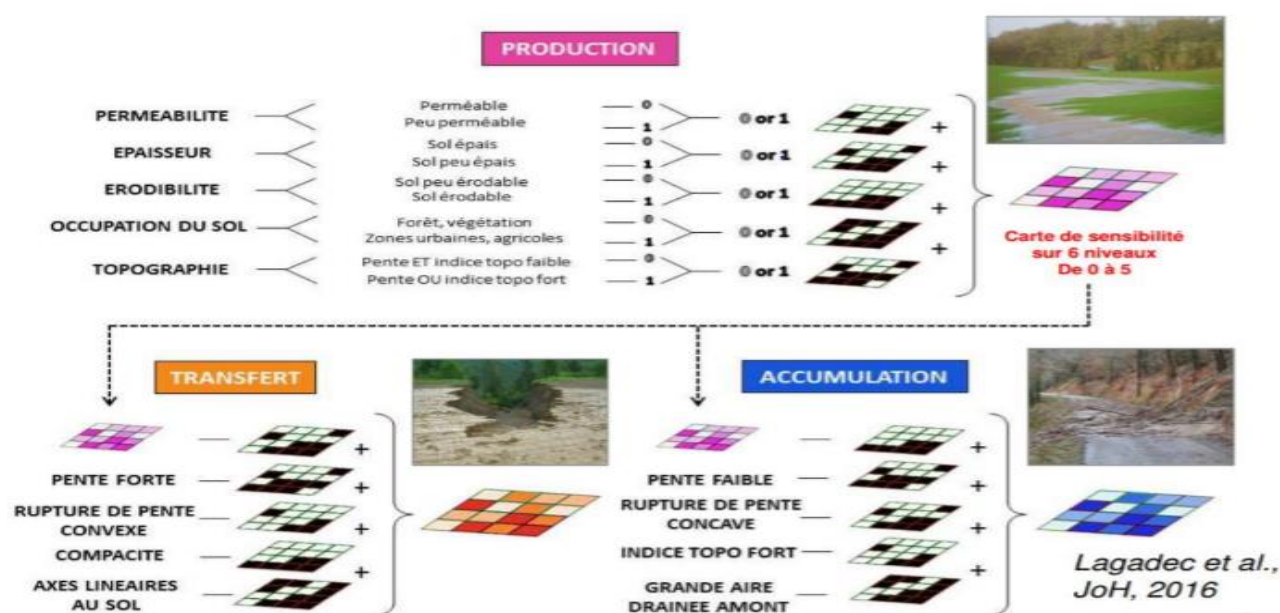
Figure 4 : Principe de l'analyse ANSETR (source : L. R. Lagadec, I. Braud, P. Breil, L. Moulin, B. Chazelle. Évaluation d'un outil cartographique pour la gestion du ruissellement pluvial intense sur les voies ferrées. Congrès Lambda Mu 21 " Maîtrise des risques et transformation numérique : opportunités et menaces ", Oct 2018, Reims, France. ffhal-02072678f).
