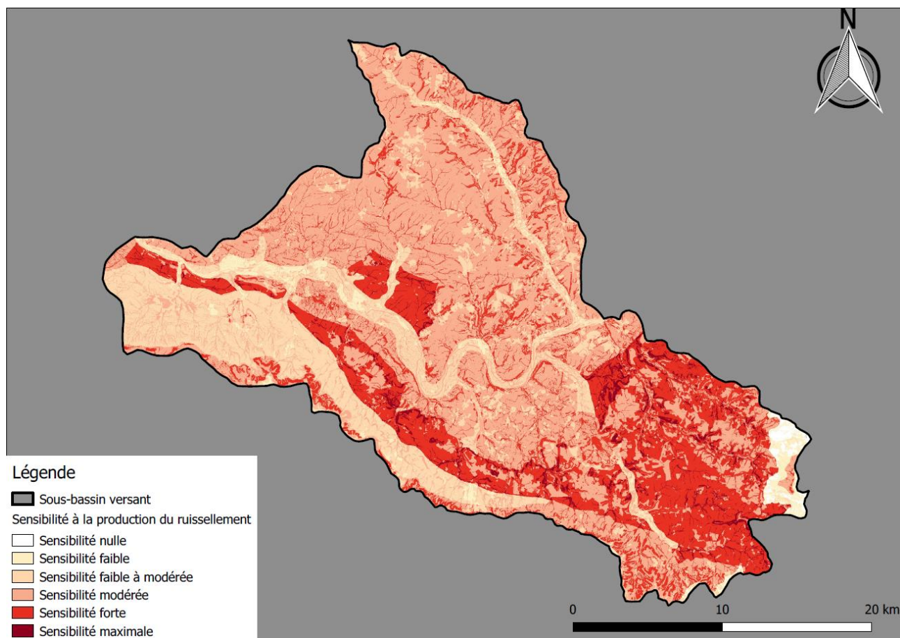
Figure 11 : Exemple de CAP sur un sous bassin versant
