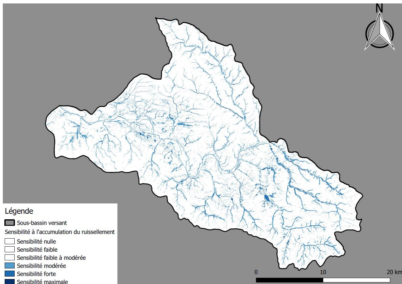
Figure 24 : Exemple de CAC sur un sous bassin versant
