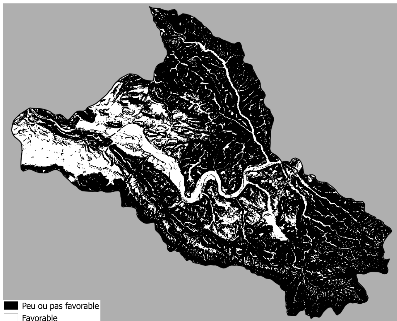
Figure 21 : Exemple de cartographie binarisée des pentes faibles sur un sous bassin versant
