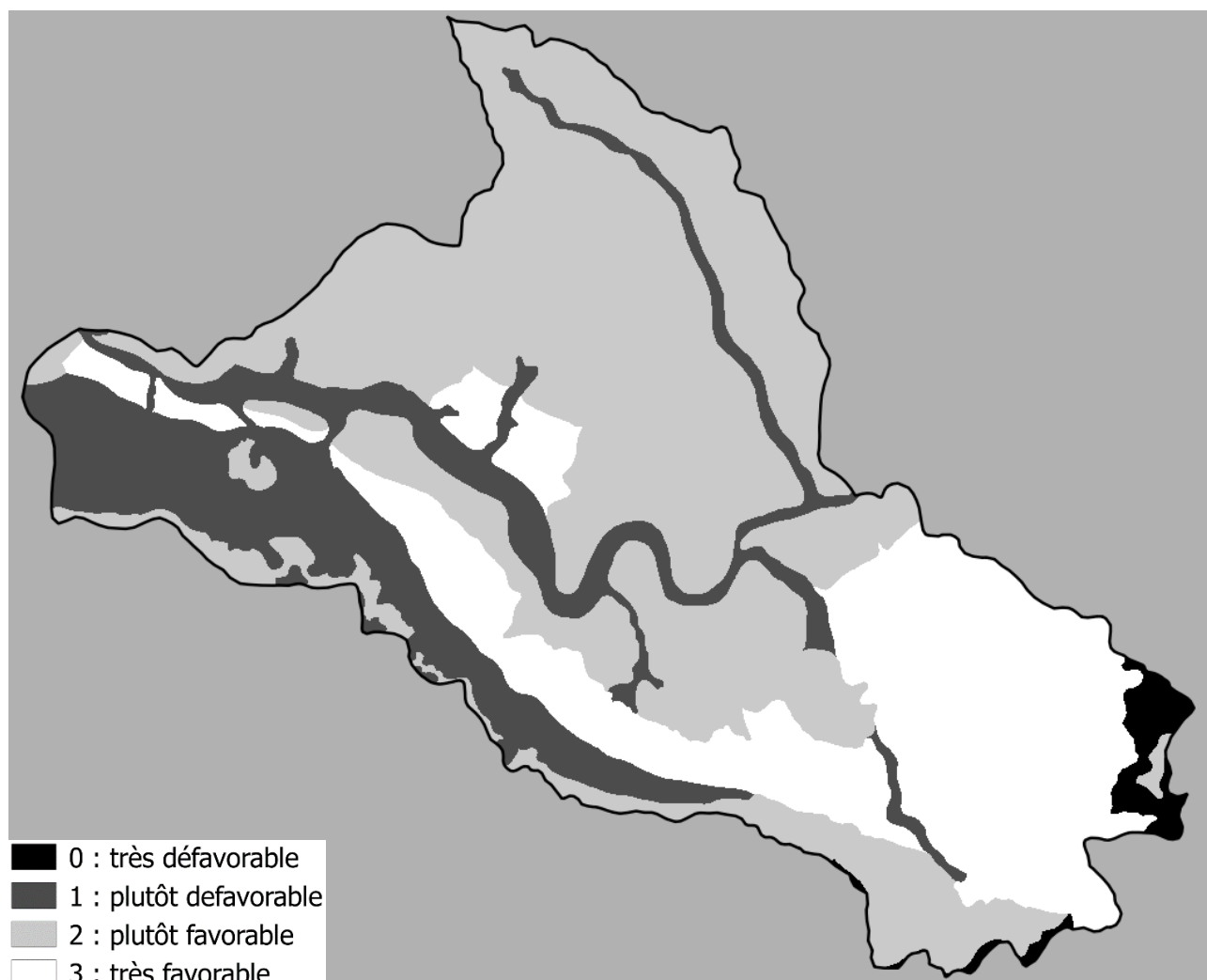
Figure 6 : Exemple de cartographie des paramètres géologiques binarisés et additionnés sur un sous bassin versant
