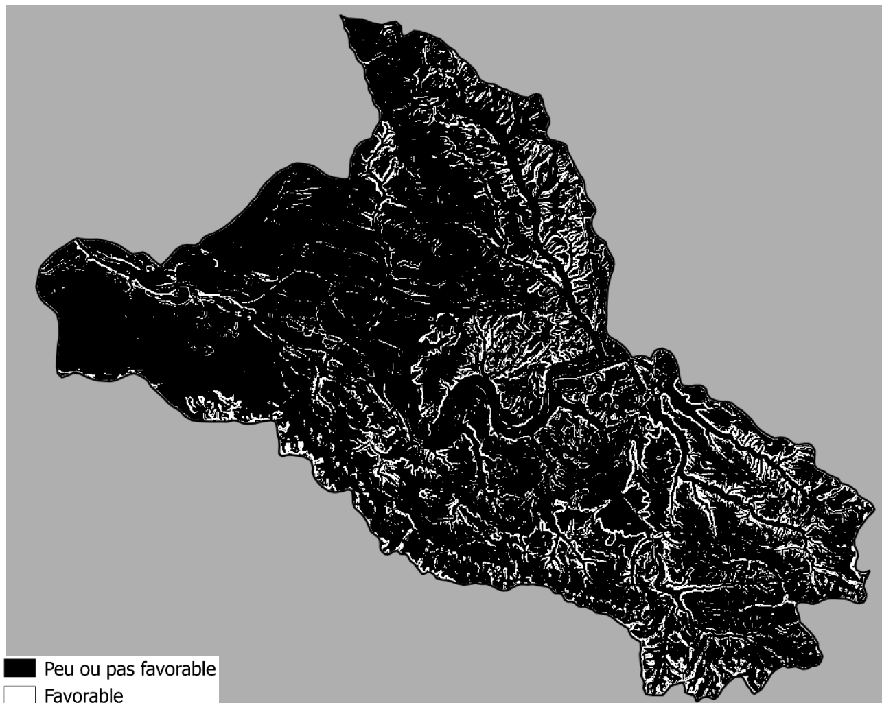
Figure 16 : Exemple de cartographie binarisée des ruptures de pente pour la CAT sur un sous bassin versant
