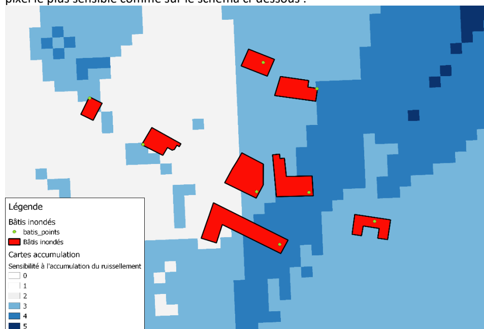
Figure 26 : Calage manuel des points représentant les bâtis inondés.
