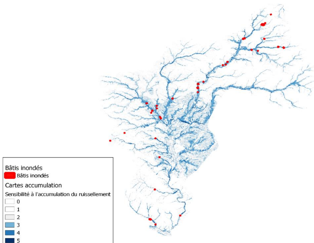
Figure 27 : Localisation des bâtiments sur la CAC calée
