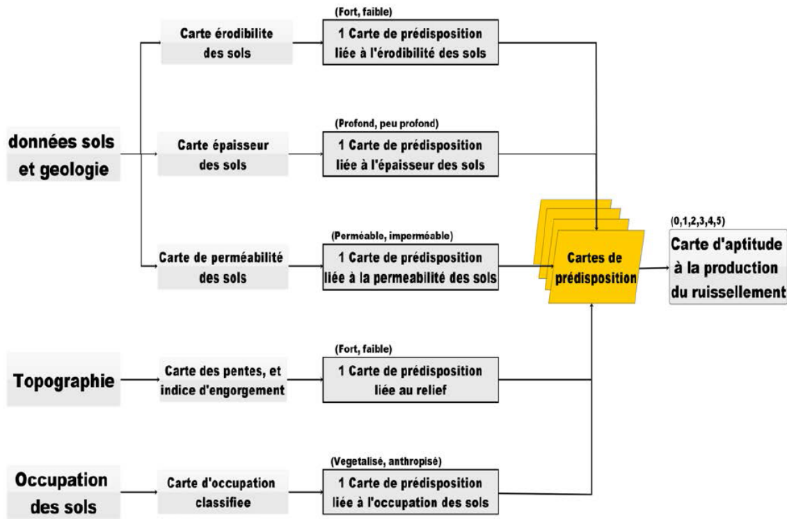
Figure 5 : Etablissement de la CAP (source : DEHOTIN J., BREIL P. Projet IRIP : Rapport technique Cartographie de l'aléa ruissellement. Note Méthodologique. Juillet 2011 ; p19)
