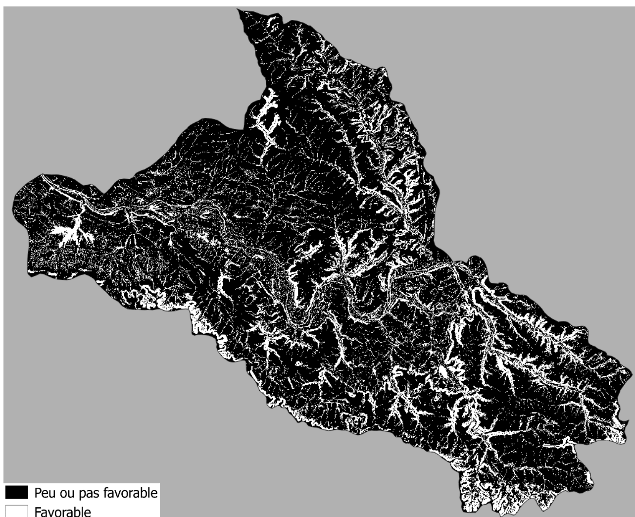
Figure 9 : Exemple de cartographie binarisée du relief sur un sous bassin versant
