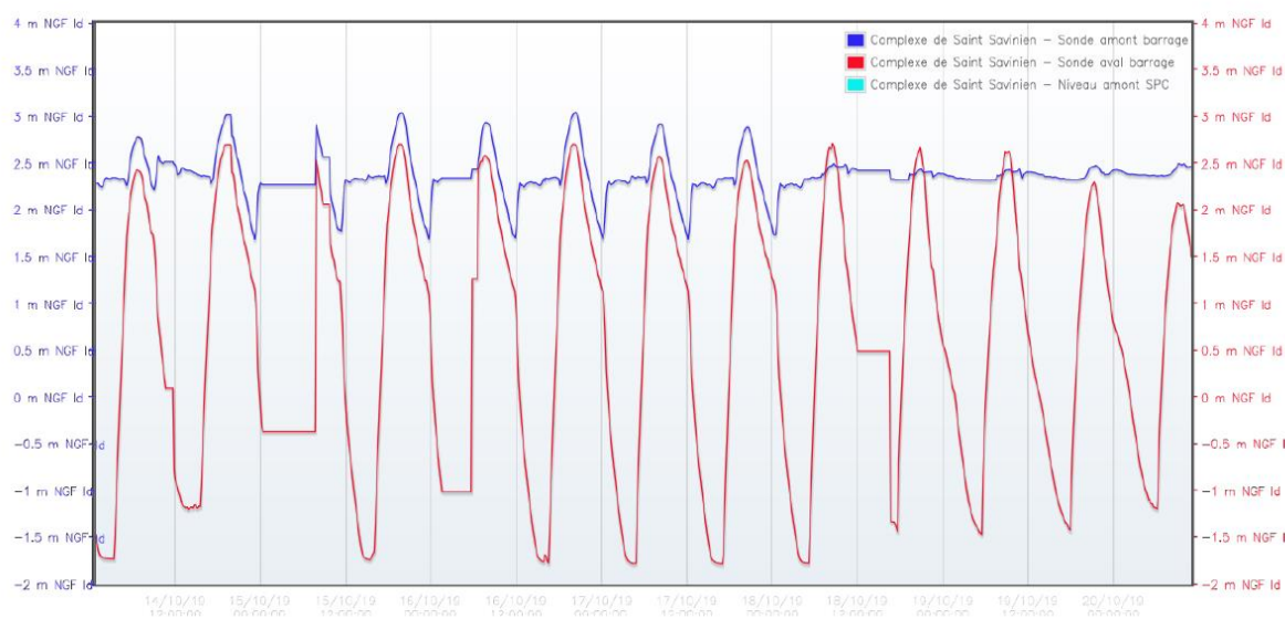
Figure 58 : niveau d'eau sonde amont et aval du barrage
