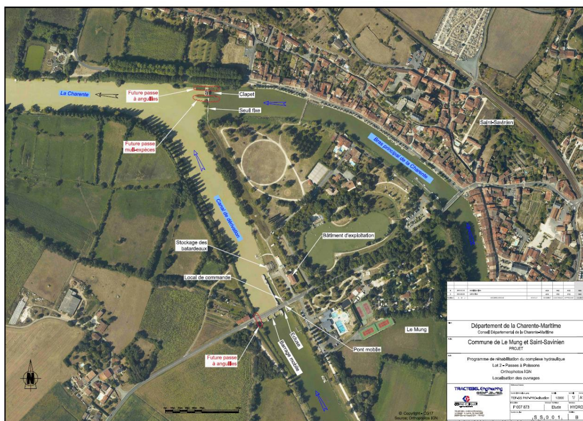
Figure 50: Vue aérienne des projets de passes-à-poissons (extrait du Rapport de maîtrise d'œuvre pour le franchissement piscicole, projet, Tractebel Engie, CD 17, 2016 ).
