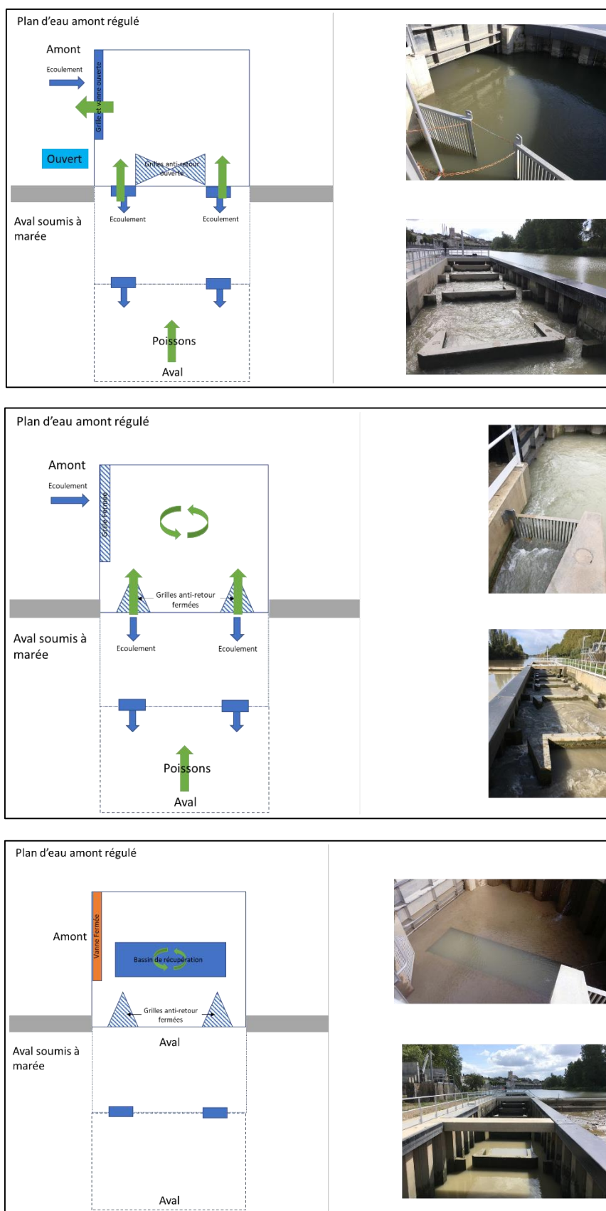
Figure 56: Schémas du fonctionnement du piège (réalisation François ALBERT pour COPIL CMCS)
