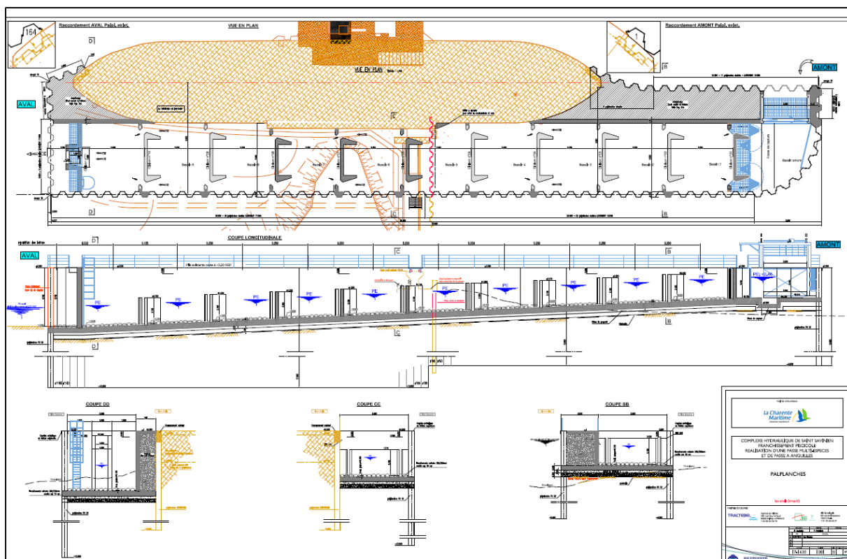
Figure 55: Plan d'exécution de la passe multi-espèces (Plan EXE, CD17 Verchéenne).
