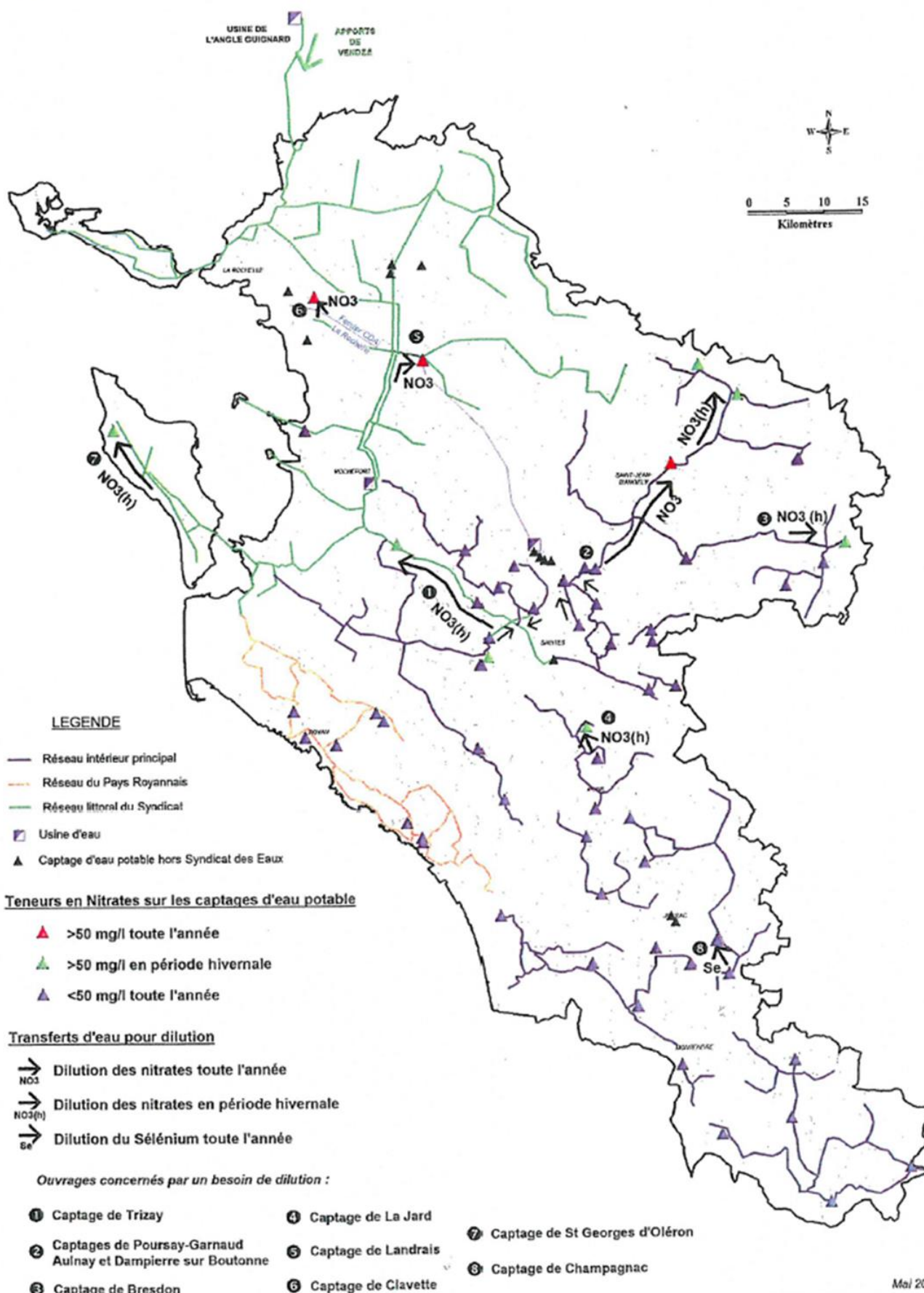
Figure 32 : Représentation du transfert entre captages AEP
