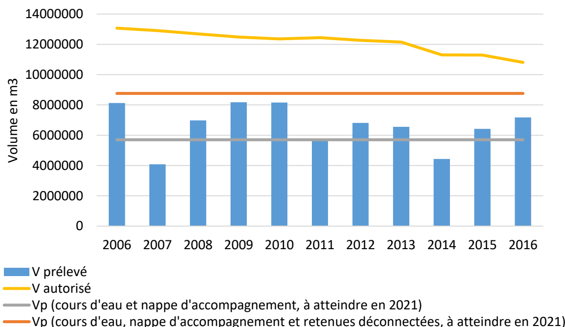
Comparaison entre volumes prélevés, volumes prélevables et volumes autorisés
