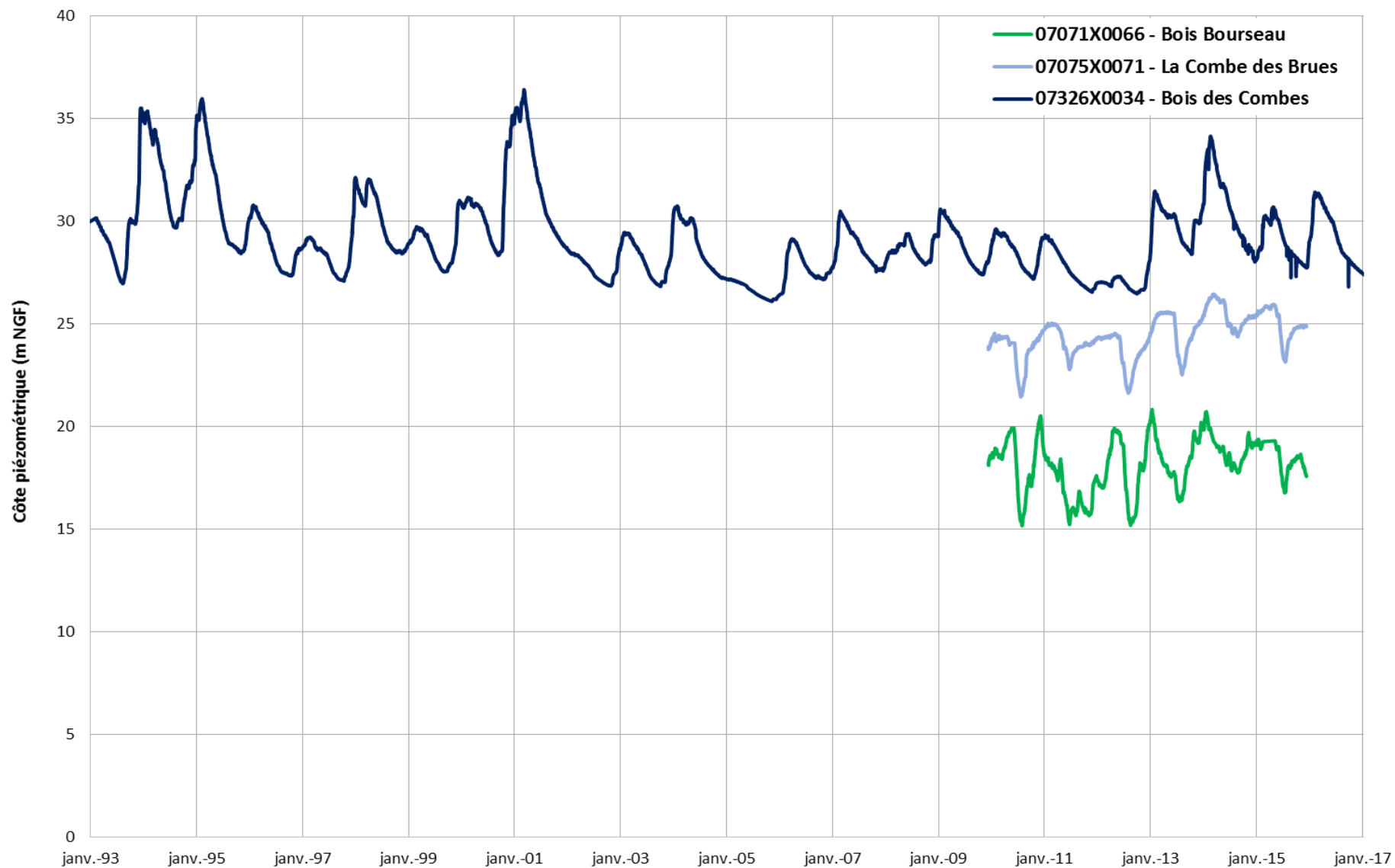
Chroniques piézométriques de la nappe du Cénomanién
