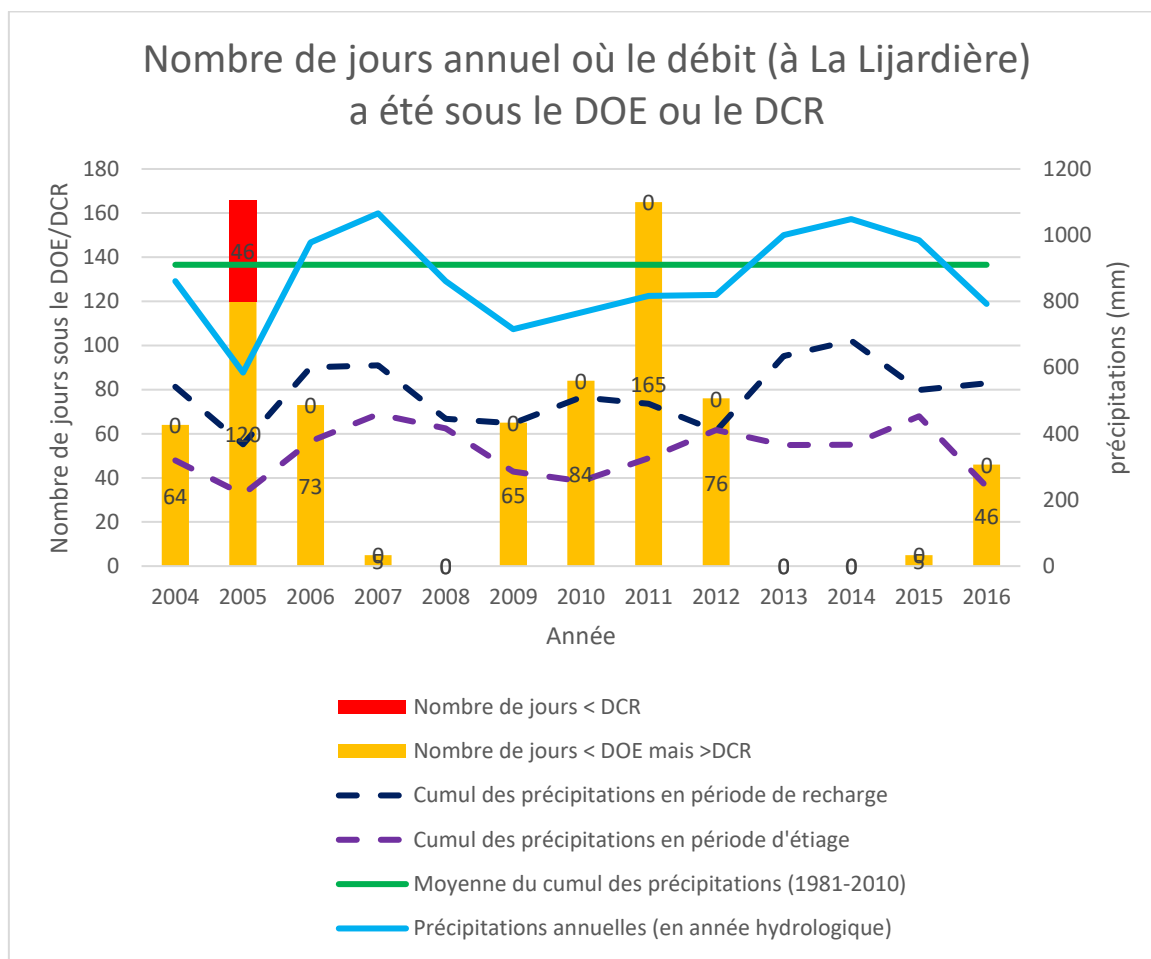
Figure 14 : Nombre de jours où le débit à la Lijardière était sous le DOE ou le DCR Source banque hydro.
