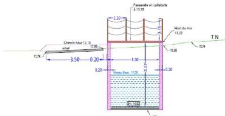
Profil en long de la passe à bassin
