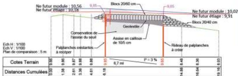
Coupe AA' (état futur)
