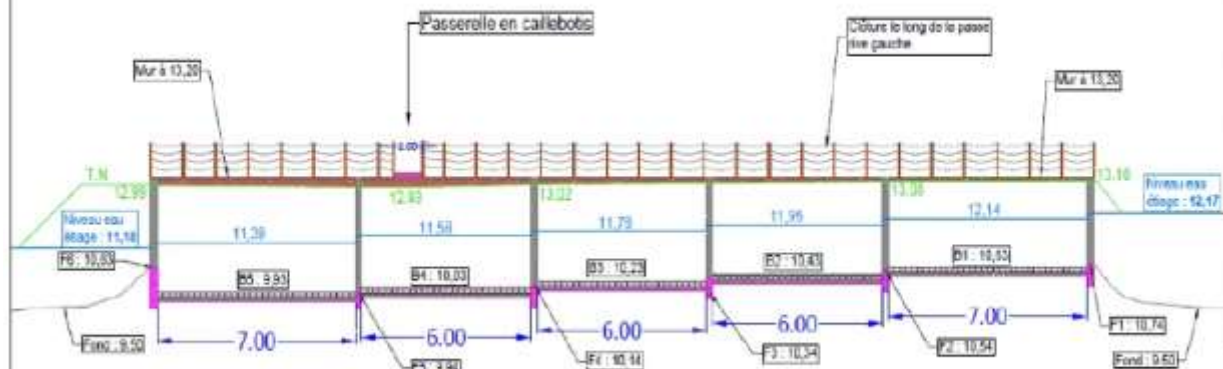
Profil en long de la passe à bassin
