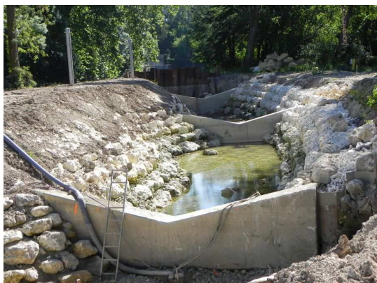
Passe à poissons de Jarnac en chantier
