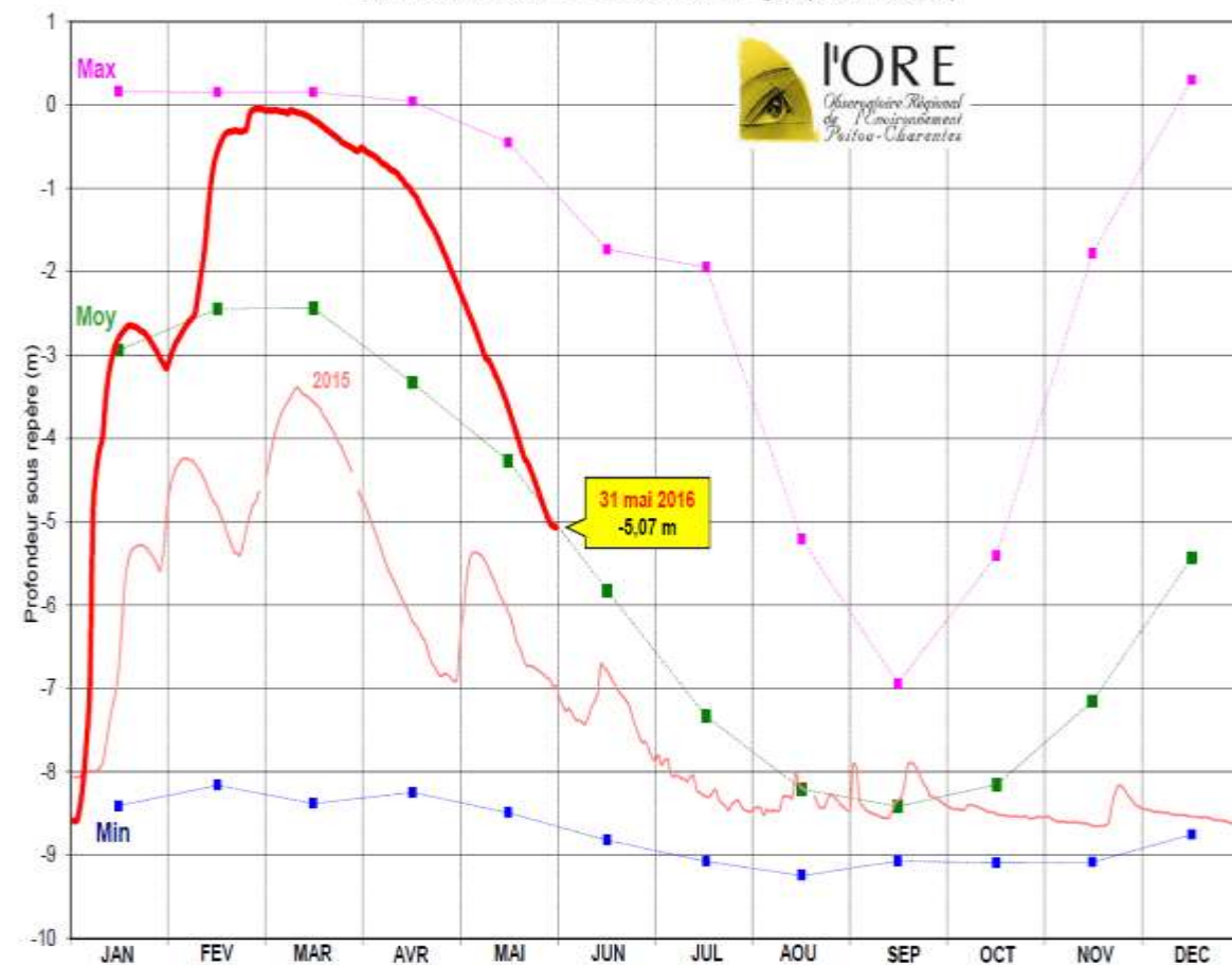
Piézomètre de RUFFEC - DOGGER LIBRE (profil période 1993-2015)
