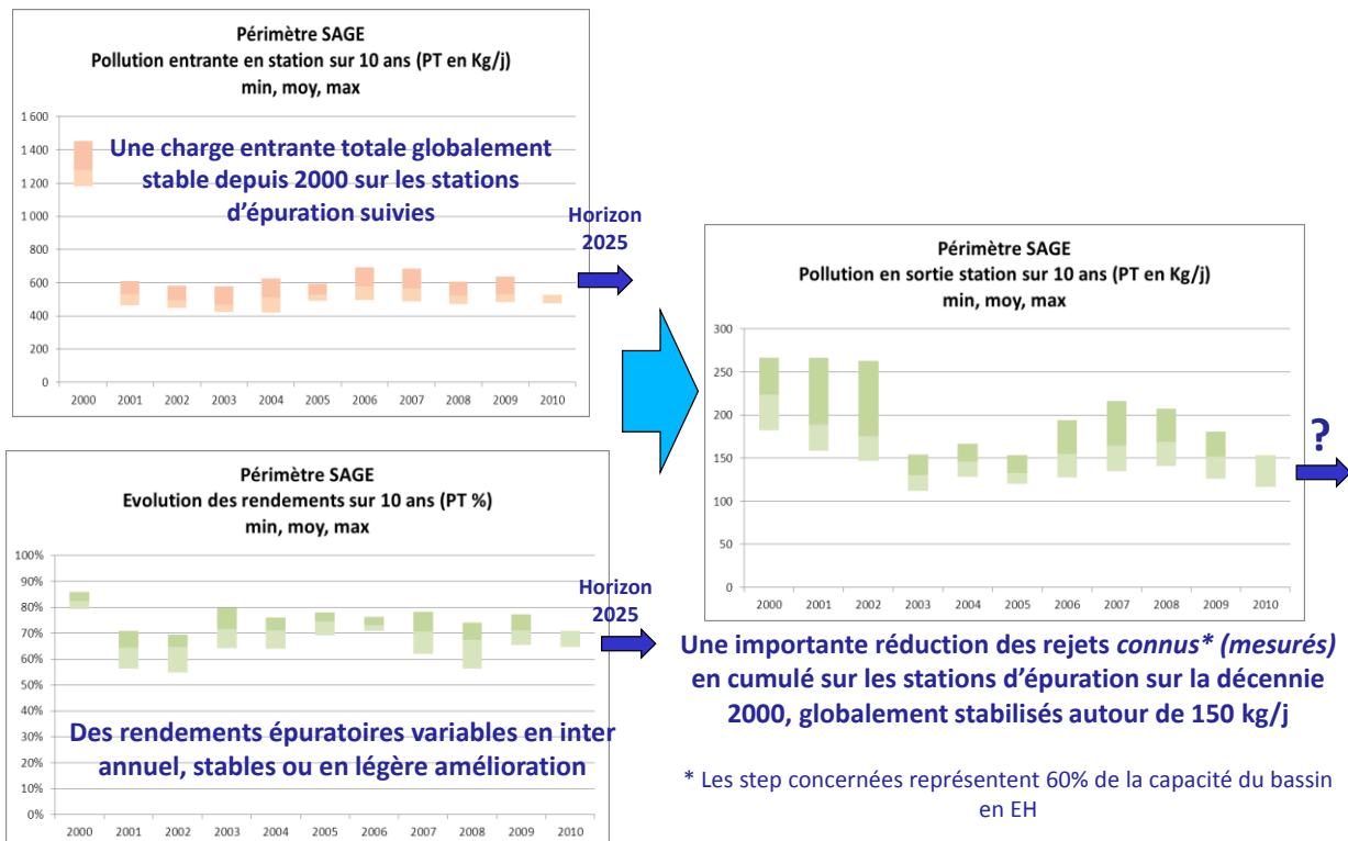
Figure 6 : Analyse de l'évolution 2000-2010 des charges d'eaux usées à traiter sur le Bassin Charente, et des performances épuratoires (sur le paramètre phosphore total )
