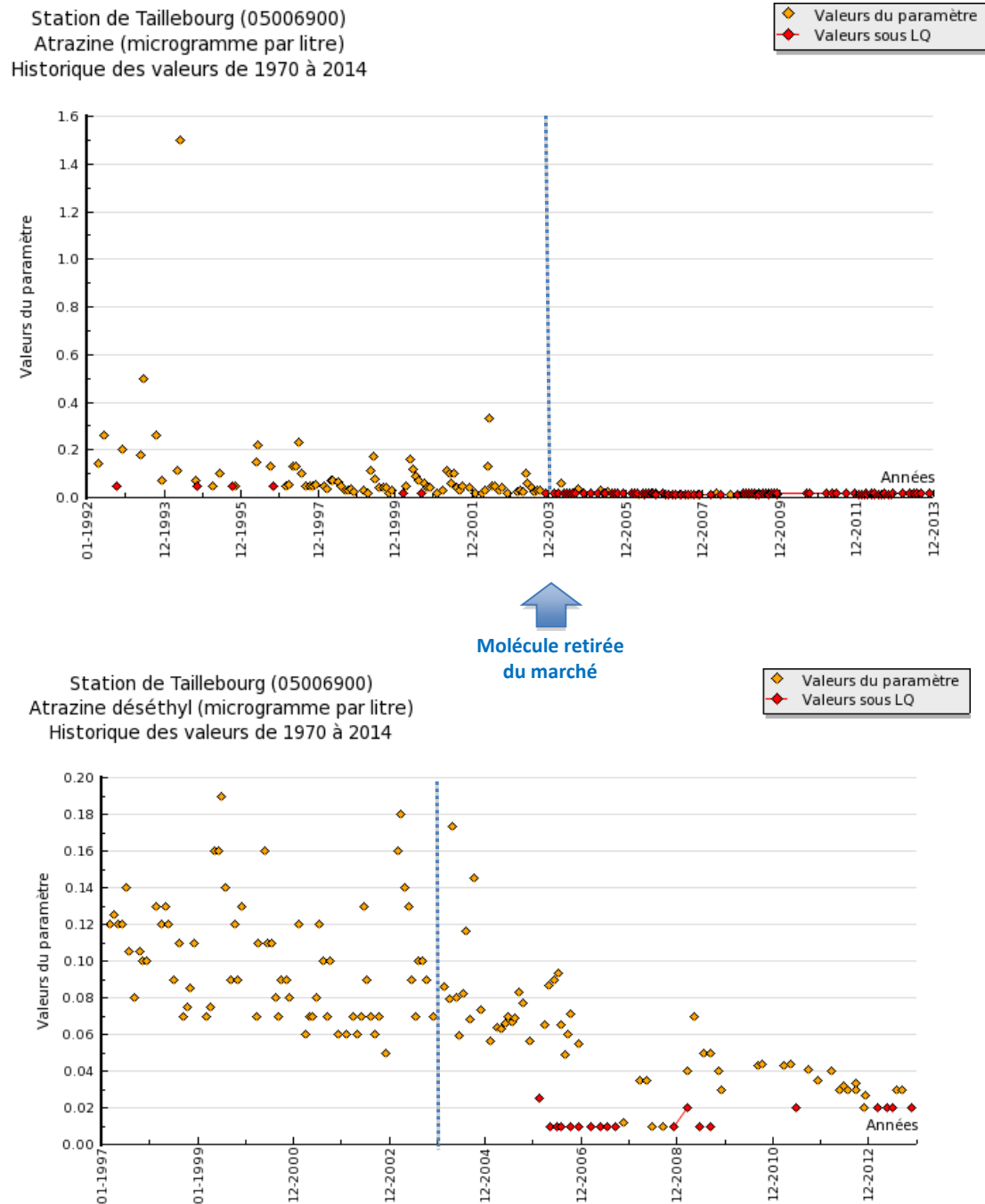
Figure 28 : Evolution de l'atrazine et son dérivé dans les eaux du fleuve Charente sur l'aval du bassin (Taillebourg), 1992-2013
