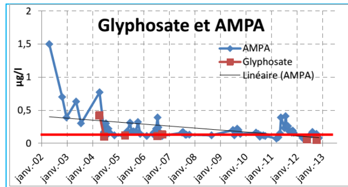
Figure 29 : Evolution des concentrations de glyphosate et d'AMPA sur le fleuve Charente (eaux captées à Coulonge) 7
