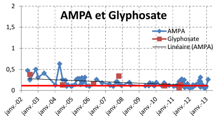
Figure 30 : Evolution des concentrations de glyphosate et d'AMPA au captage de St Hippolyte
