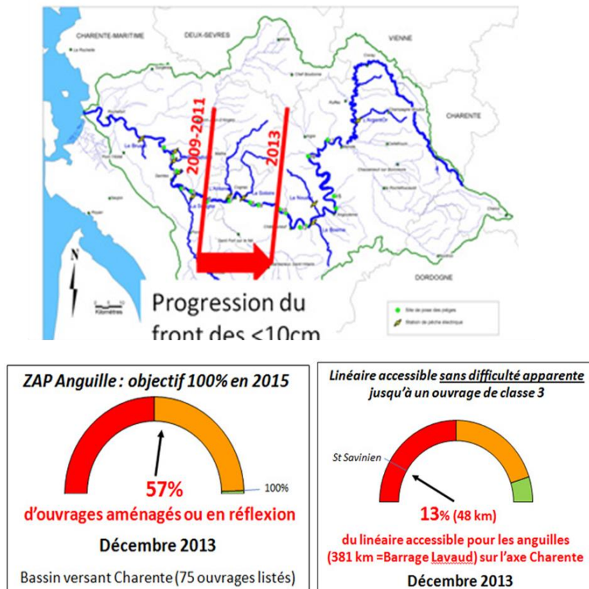
Figure 36. Indicateurs de progression du front de migration de l'Anguille (Source : cellule migrateurs Charente, 2014)
