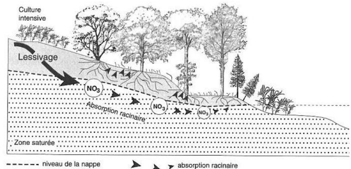
Fig. 6 : Circulation de nutriments dans les eaux du sous-écoulement du prélèvement racinaire. (D'après Ruffinoni, 1993, modifié).
