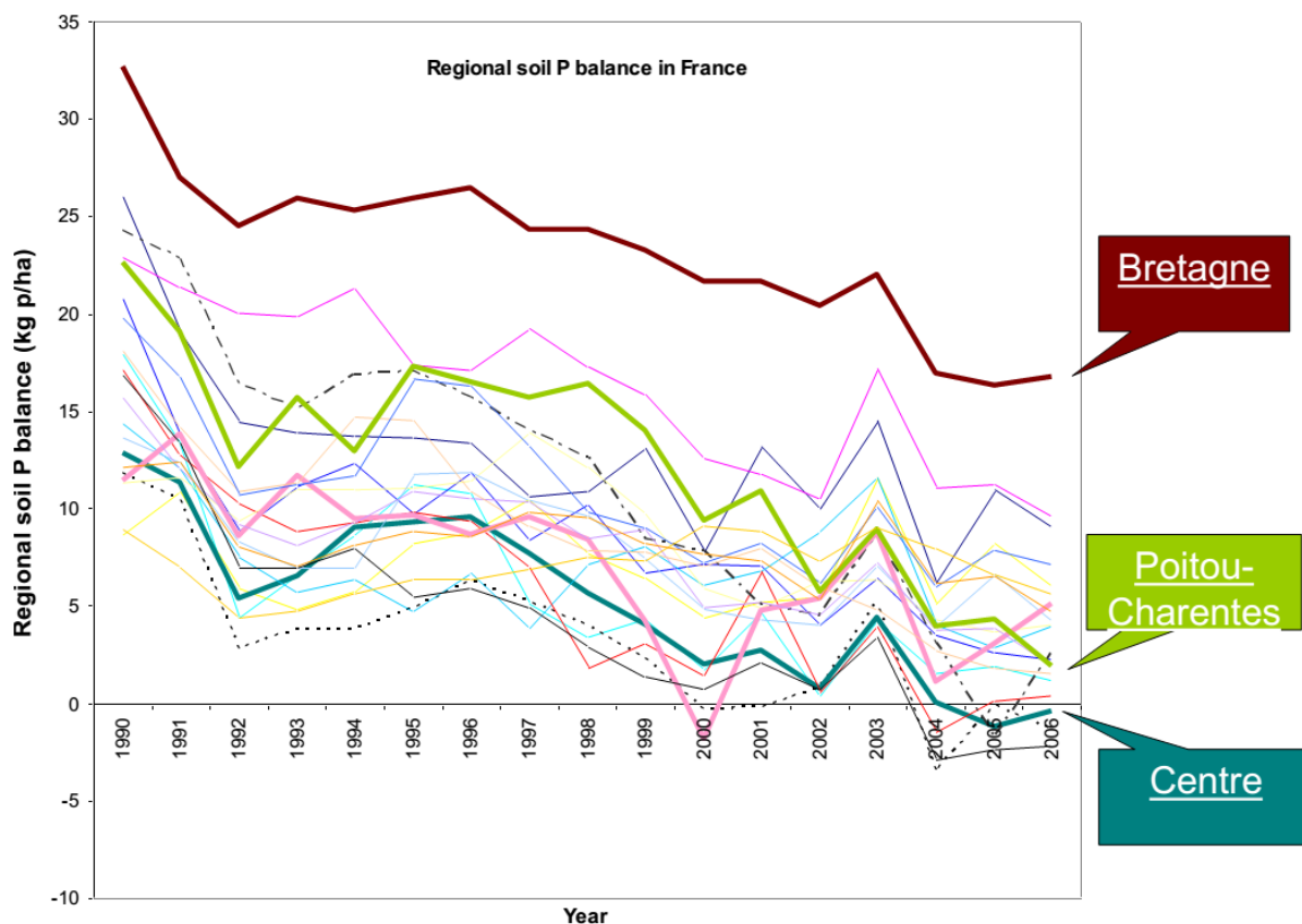
Bilan P des sols des 21 régions françaises entre 1990 et 2006 en kg P ha -1 an -1 (in Kalimuthu, 2012)
