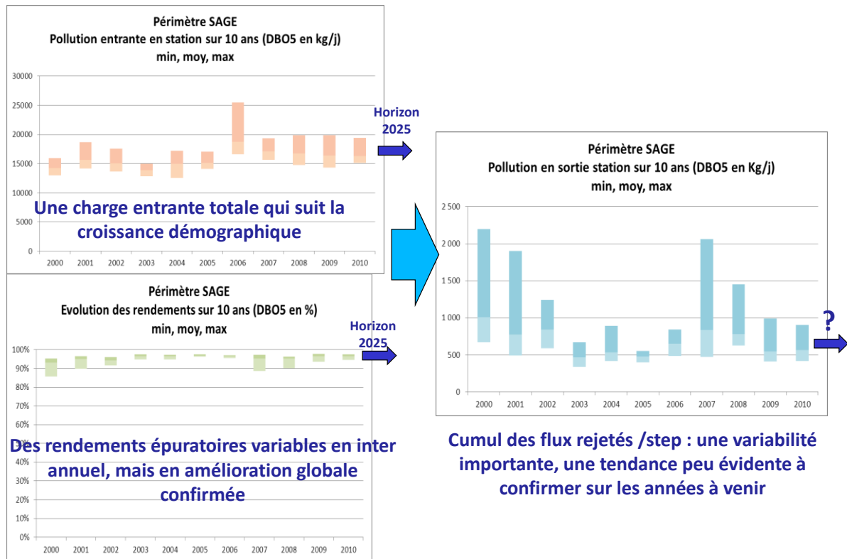
Figure 5 : Analyse de l'évolution 2000-2010 des charges d'eaux usées à traiter sur le Bassin Charente, et des performances épuratoires (sur le paramètre DBO5 : indicateur de la matière organique biodégradable dans l'eau).
